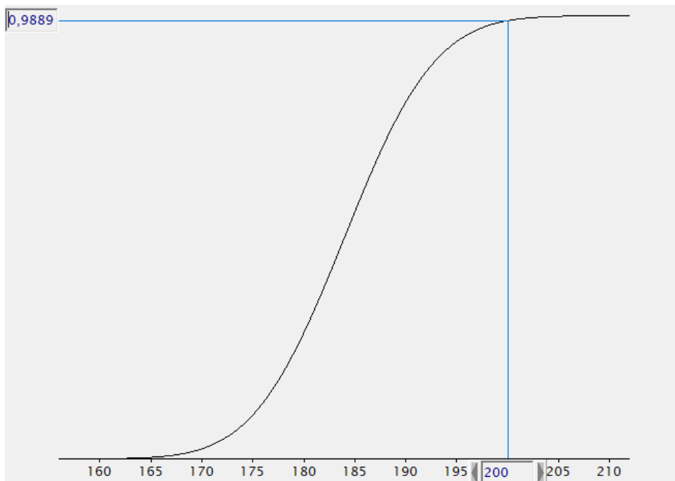
Figuur 9. De plek waar een lengte van 200 cm past in een normaalverdeling van lengtes van Nederlandse mannen. Deze keer afgebeeld in een cumulatieve verdeling.
