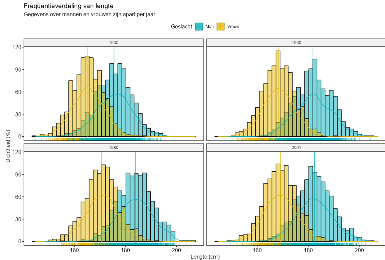
Figuur 50. Verdeling man en vrouw per jaar.
