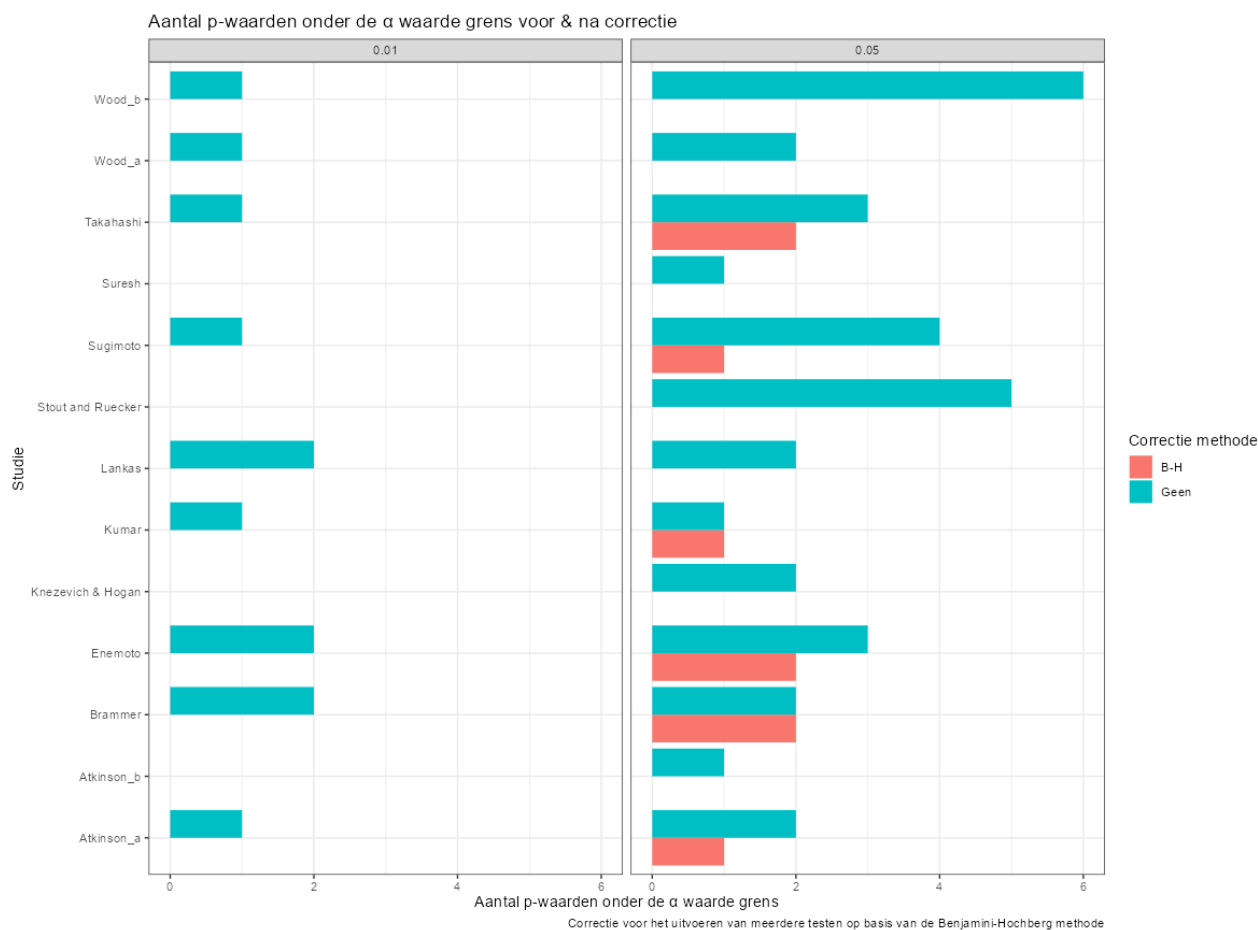
Figuur 80. Per studie en geslacht het aantal toetsen dat onder een gespecificeerde grenswaarde viel met of zonder correctie methode. Dit zijn resultaten zoals door Portier gerapporteerd.
