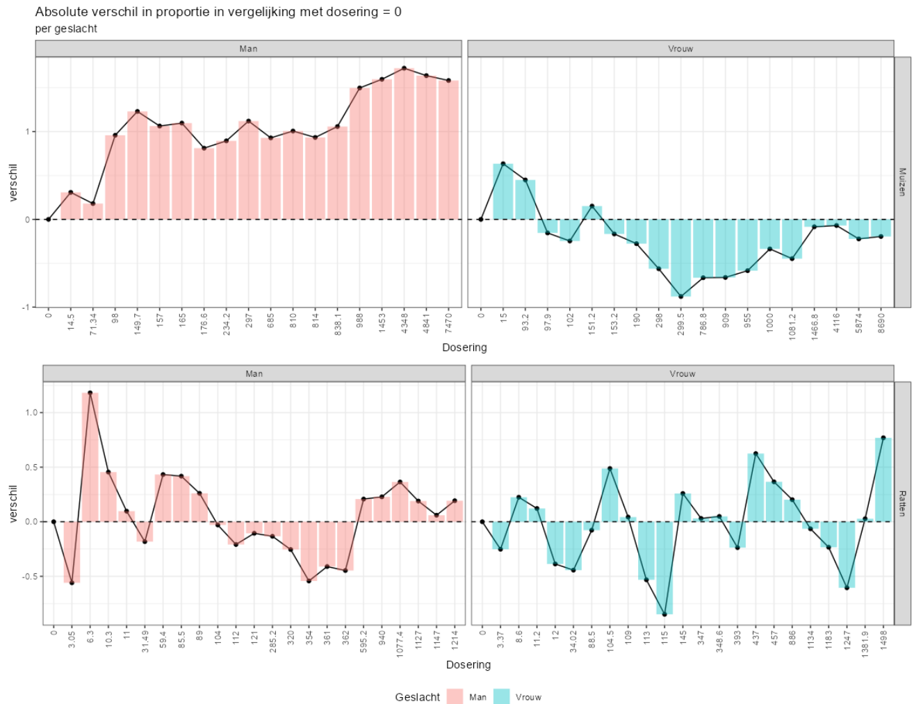
Figuur 64. Absolute verschil in proporties tussen de nuldosering en de andere doseringen per geslacht én diersoort.
