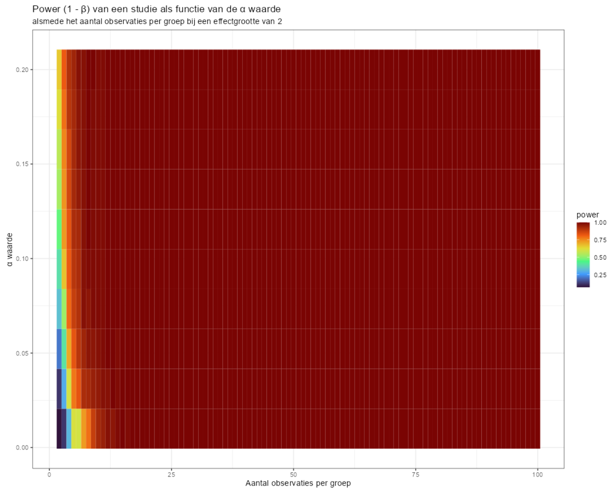
Figuur 37. De relatie tussen de \alpha waarde en de power ( 1 - \beta ) van een studie bij verschillende aantallen observaties per groep. Omdat de effectgrootte zo groot is (2) maakt de keuze voor de \alpha waarde eigenlijk niet meer uit.
