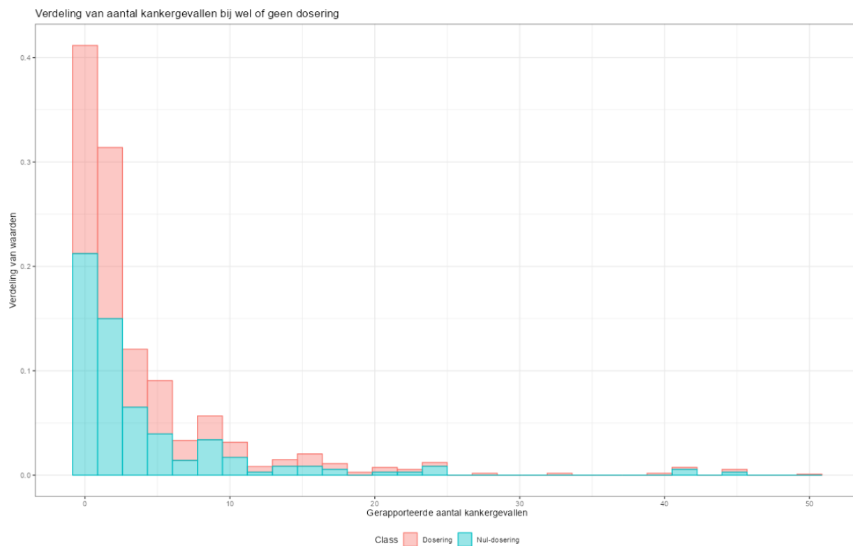
Figuur 157. Verdeling van het aantal kankergevallen per nul-dosering en dosering waarbij dosering is samengevoegd tot één groep.
