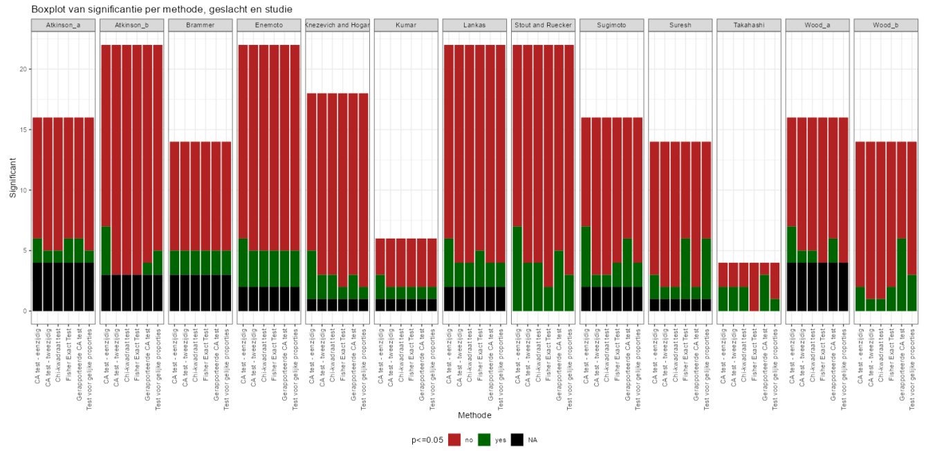
Figuur 73. Boxplot die per methode en per studie het aantal significante resultaten laat zien voor p \leq 0.05 .
