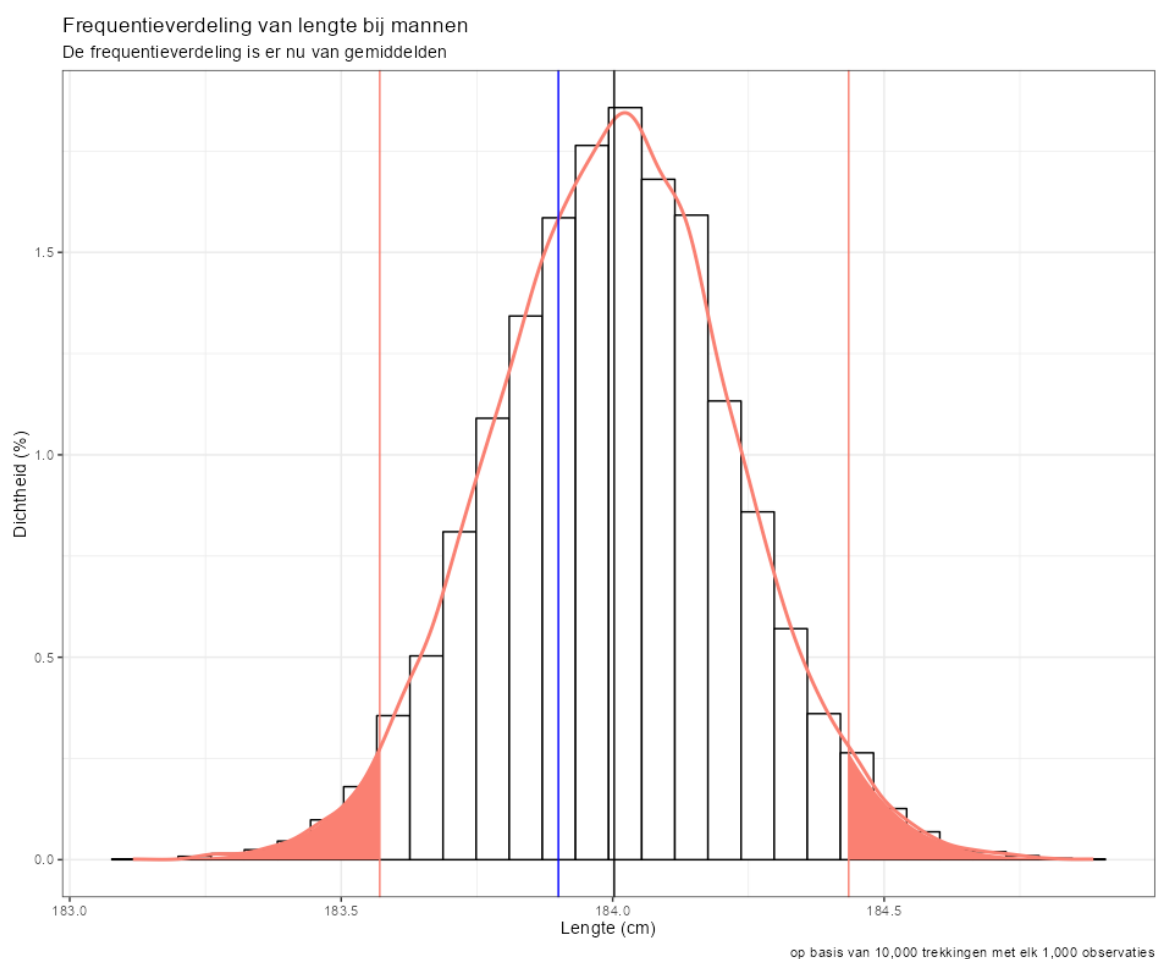
Figuur 26. Gesimuleerde verdeling van gemiddeldes. De blauwe lijn is één willekeurig gekozen gemiddelde. De zwarte lijn laat het gemiddelde van alle gemiddeldes zien (184 cm) en de rode lijnen tonen het 95% betrouwbaarheidsinterval.
