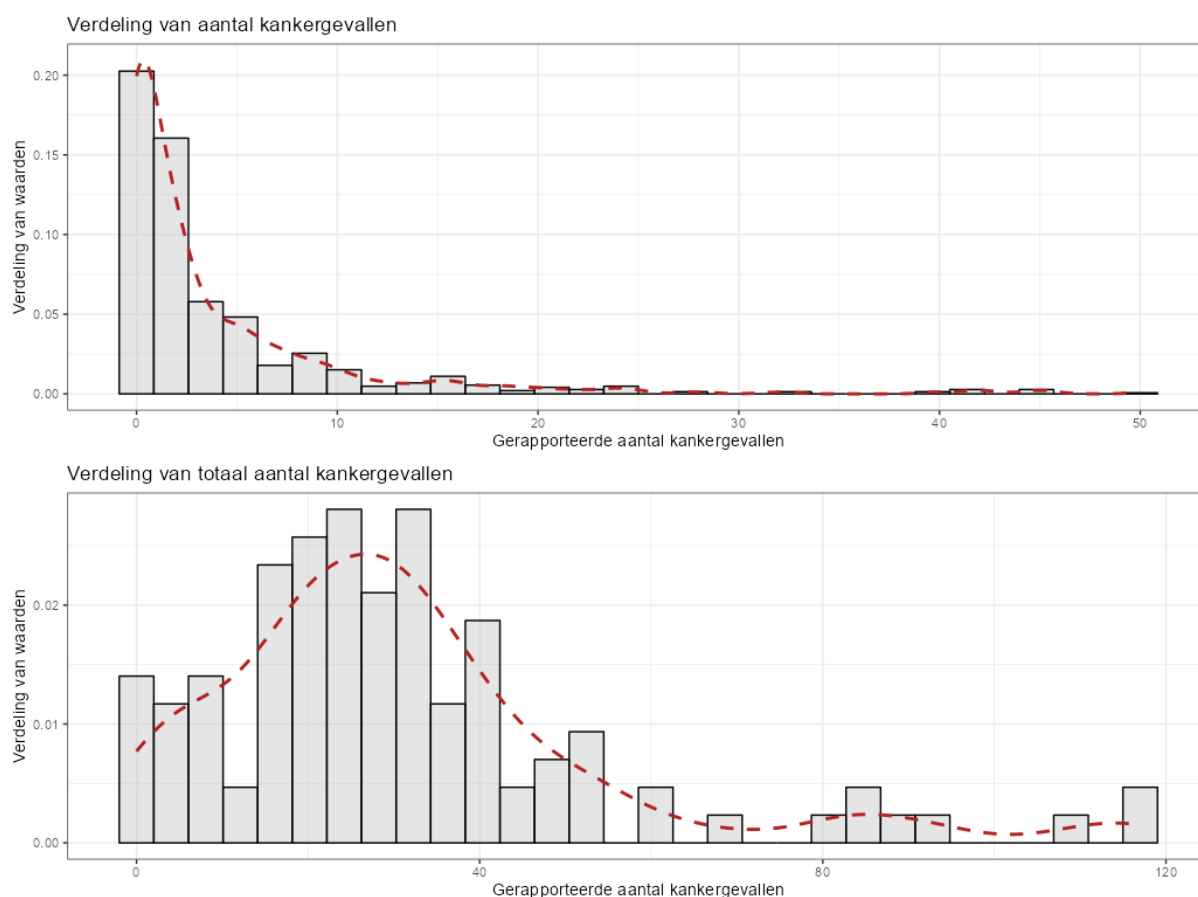
Figuur 149. Verdeling van het aantal kanker gevallen (boven, en verdeling van het totaal aantal kanker gevallen per studie, geslacht en dosering (onder).
