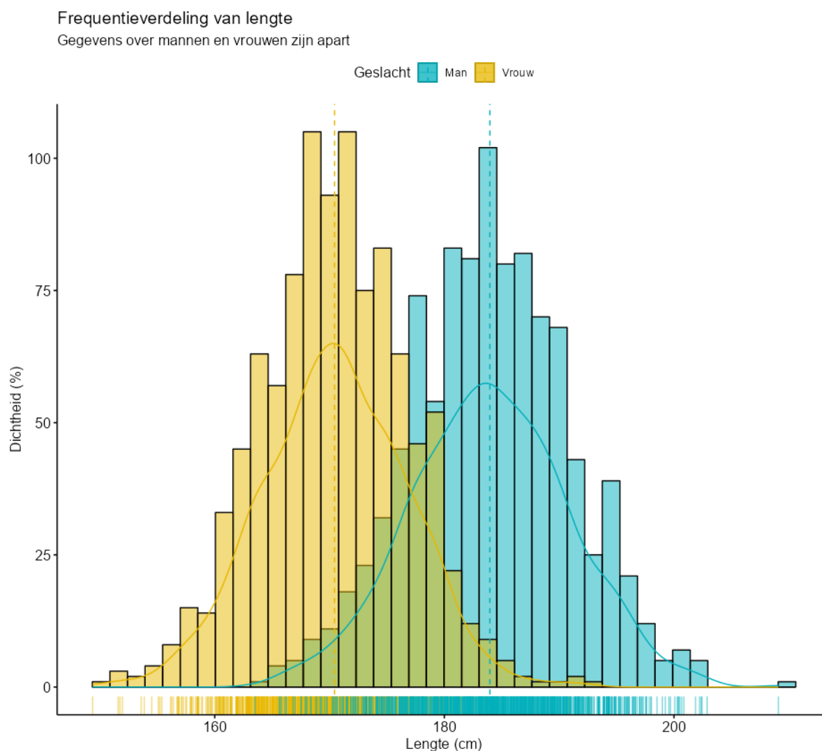
Figuur 15. De verdeling van Nederlandse mannen en vrouwen in eenzelfde grafiek. Zichtbaar zijn de verschillende pieken en de overlap. Beiden zijn van betekenis.
