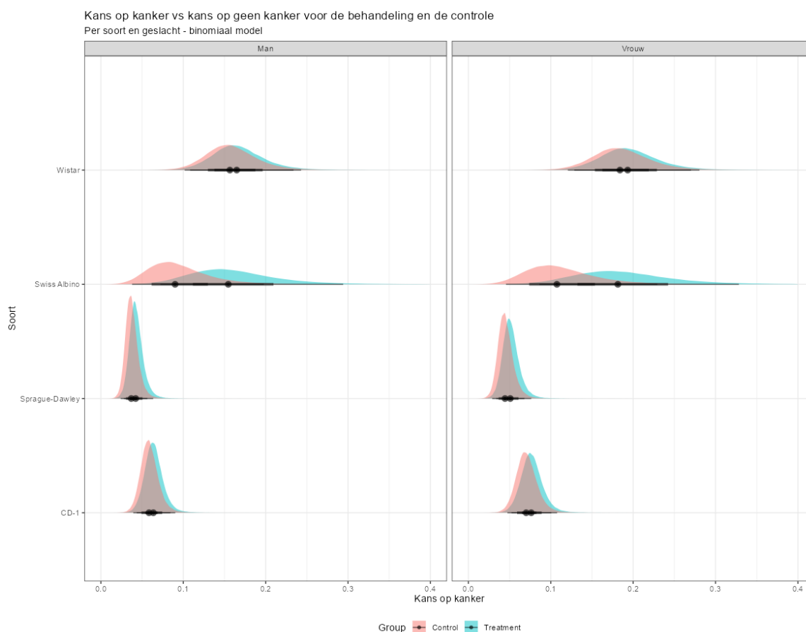
Figuur 169. De kans op kanker, berekend vanuit het model, per soort en per geslacht.
