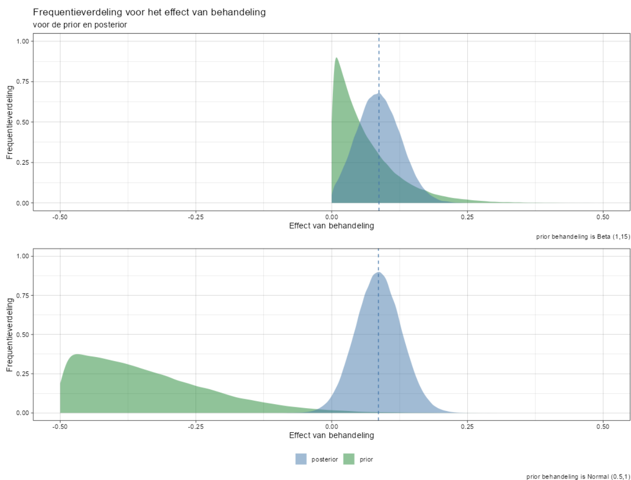
Figuur 176. De invloed van twee priors op de posterior. De Beta prior gaat er van uit dat behandeling de kans op kanker verhoogt. De normaalverdeling is een prior met de aanname dat glyfosaat de kans op kanker verkleint.
