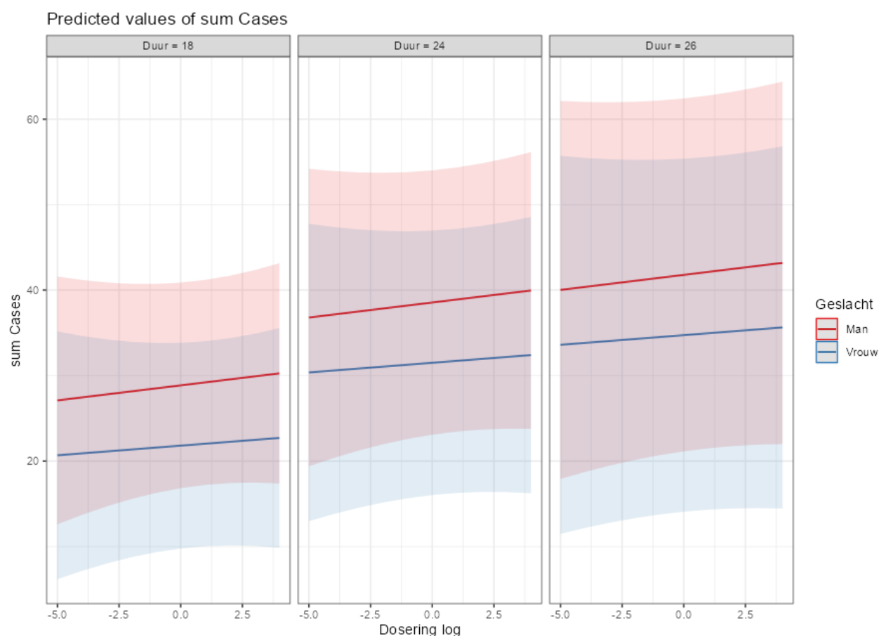
Figuur 90. Voorspellingen afkomstig van een LMM model met als y-variabele het opgeteld aantal kankergevallen ( sum Cases ). De lijn laat de voorspelde waarde zien als functie van de dosering (log schaal), geslacht en de duur van de studie. De lijnen laten de gemiddelde voorspelling zien, de band eromheen is de onzekerheid.
