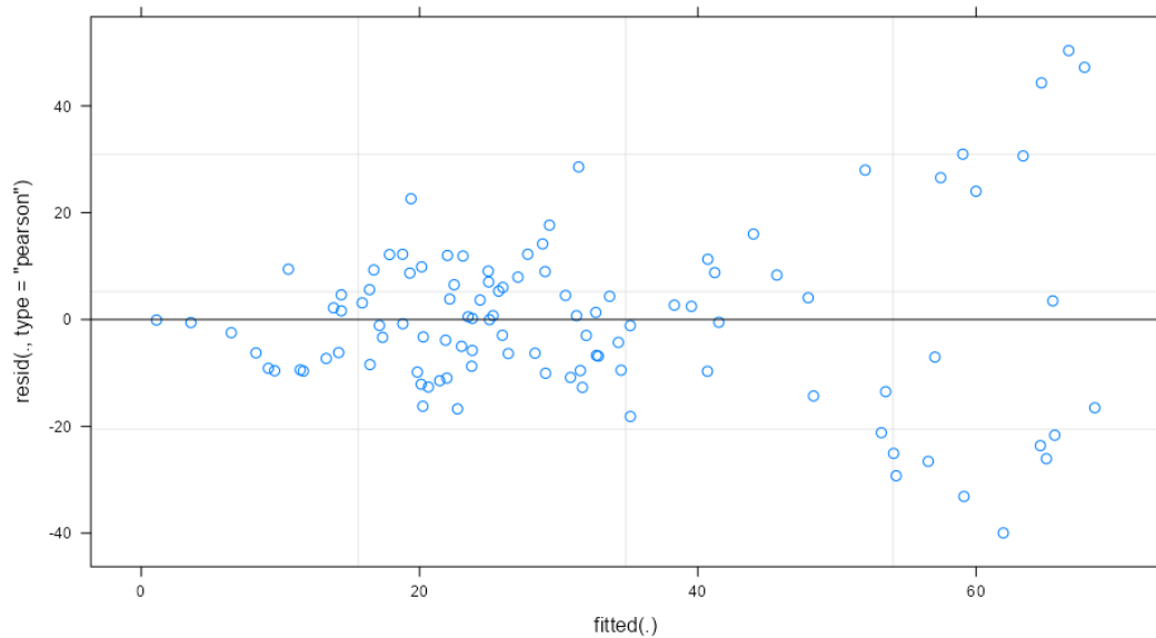
Figuur 93. Restwaarden van een LMM met natural splines. De waaier op het einde is te groot, wat maakt dat het model ook te veel te wensen overlaat.
