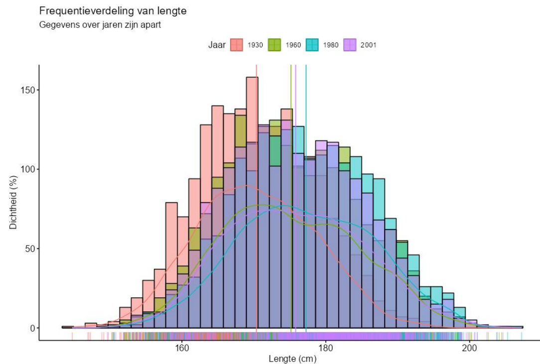
Figuur 49. Verdeling per jaar over de geslachten heen.
