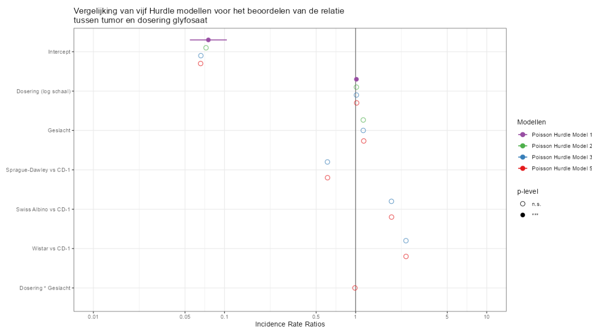
Figuur 134. Schattingen voor elke parameter in een specifiek Poisson Hurdle model.
