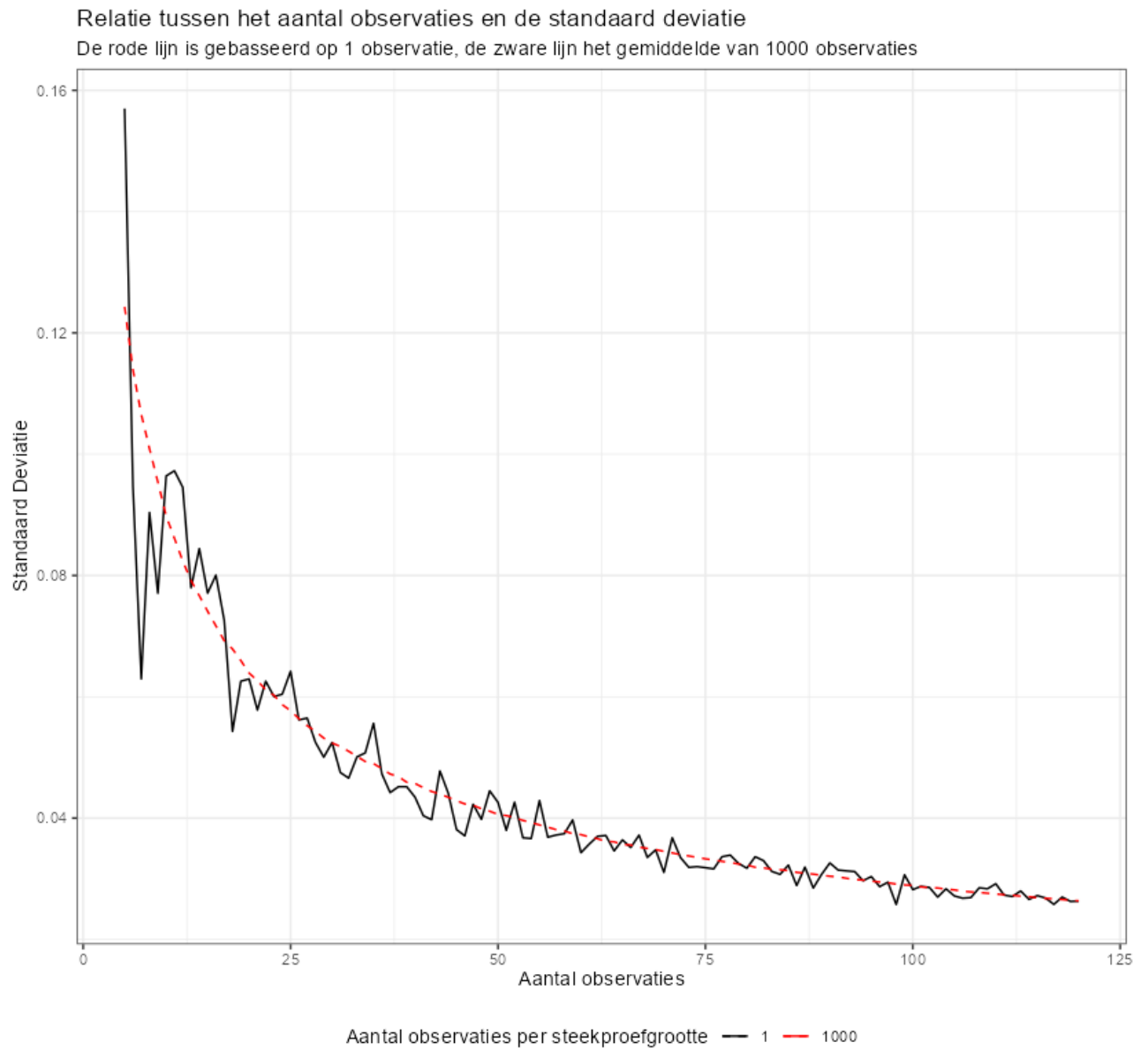
Figuur 30. Relatie tussen standaard deviatie en aantal observaties per steekproefgrootte.
