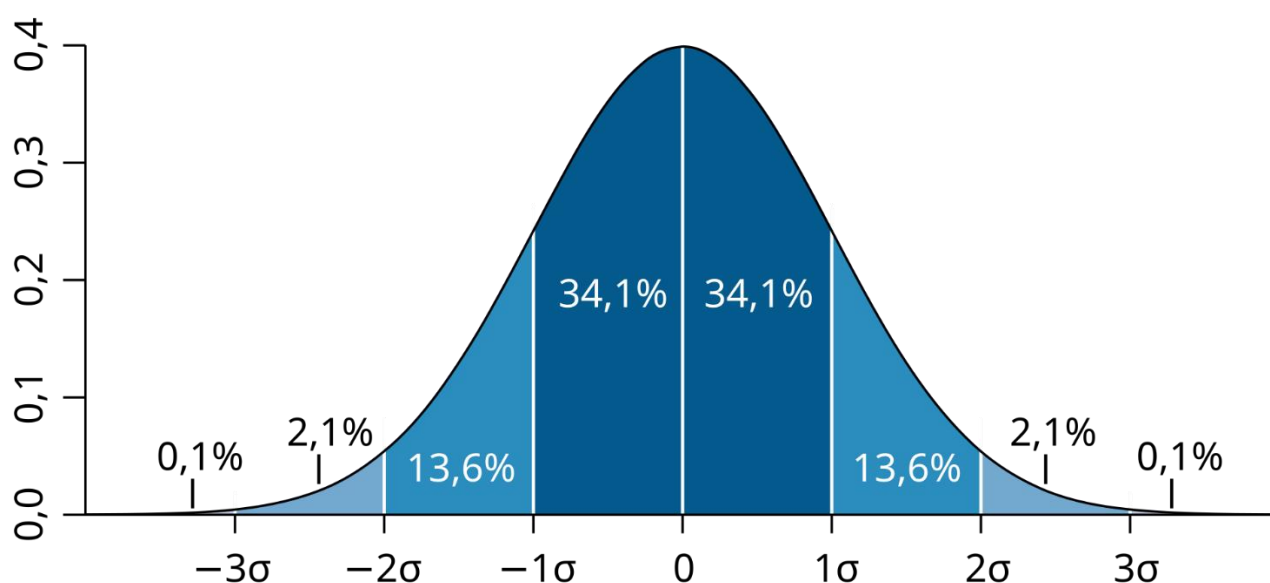
Figuur 2. De theoretische verdeling van massa in een normaalverdeling. Ongeveer 68% van de gegevens vallen binnen één standaard deviatie van het gemiddelde. Bij twee standaarddeviaties is dat ongeveer 95%.
