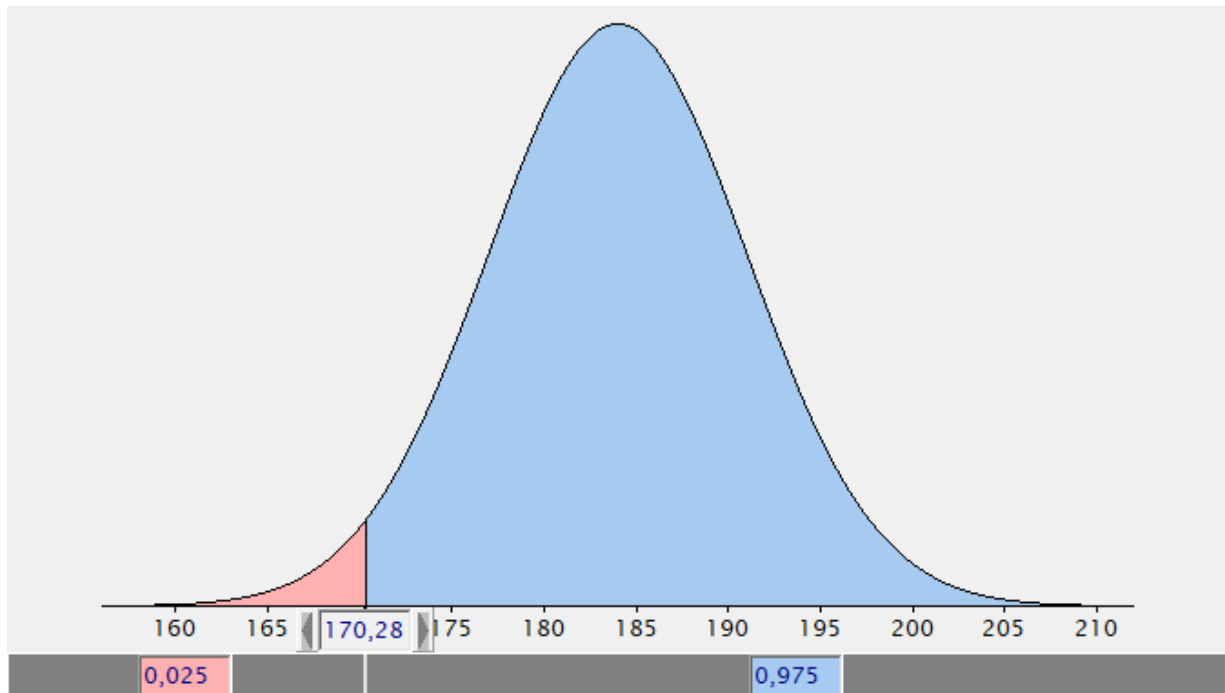
Figuur 3. De normaalverdeling met een gemiddelde van 184 cm en een standaard deviatie van 7 cm. Dit is waarschijnlijk hoe de verdeling van lengte bij de Nederlandse mannen verdeeld is.
