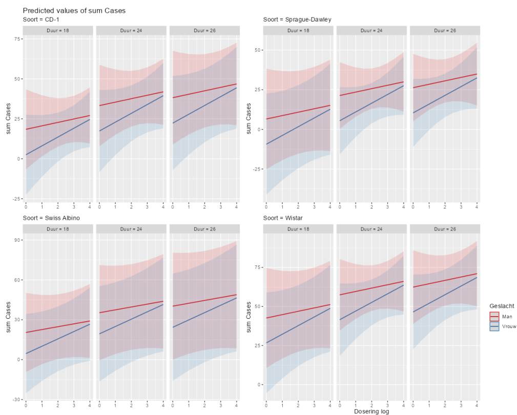
Figuur 97. Voorspellingen vanuit het model per geslacht, soort en duur. De nul-dosering is verwijderd. De relatie heeft nu een meer duidelijke richtingscoëfficiënt, maar toont nog steeds grote onzekerheden rondom deze schattingen. Dit maakt dat ook in dit model de nulhypothese niet verworpen kan worden.
