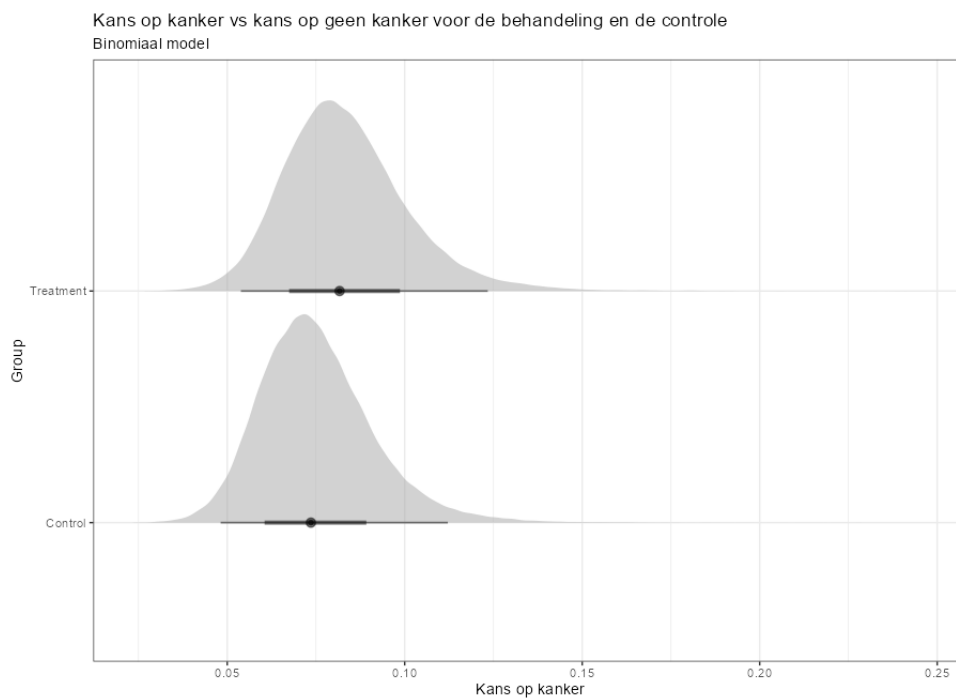
Figuur 163. Kans op kanker voor de controlegroep en de behandel (Treatment) groep.
