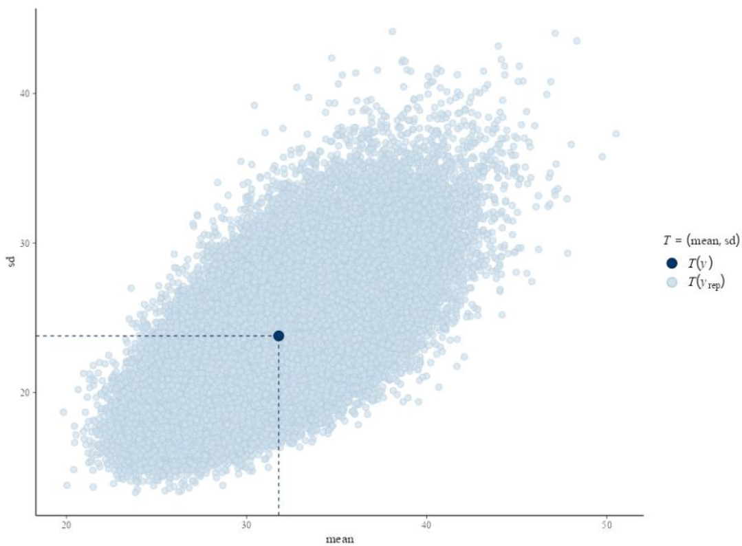
Figuur 151. De verdeling van de posterior voor een leeg hurdle model (lichte bollen), en de verdeling van de geobserveerde tumorgevallen (donkere bol).
