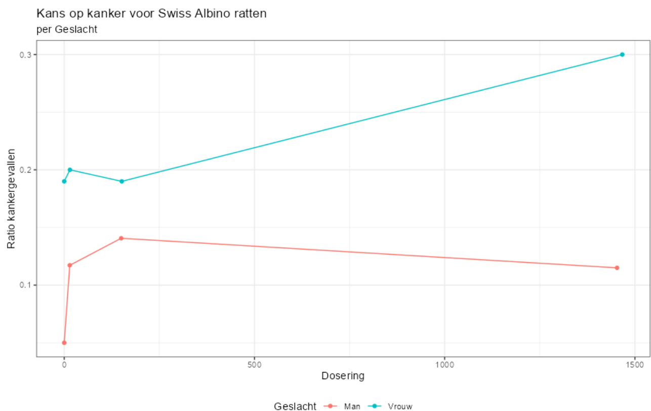
Figuur 171. Kans op kanker voor Swiss Albino ratten per geslacht – gebaseerd op de studie van Kumar die de enige studie is met Swiss Albino ratten.
