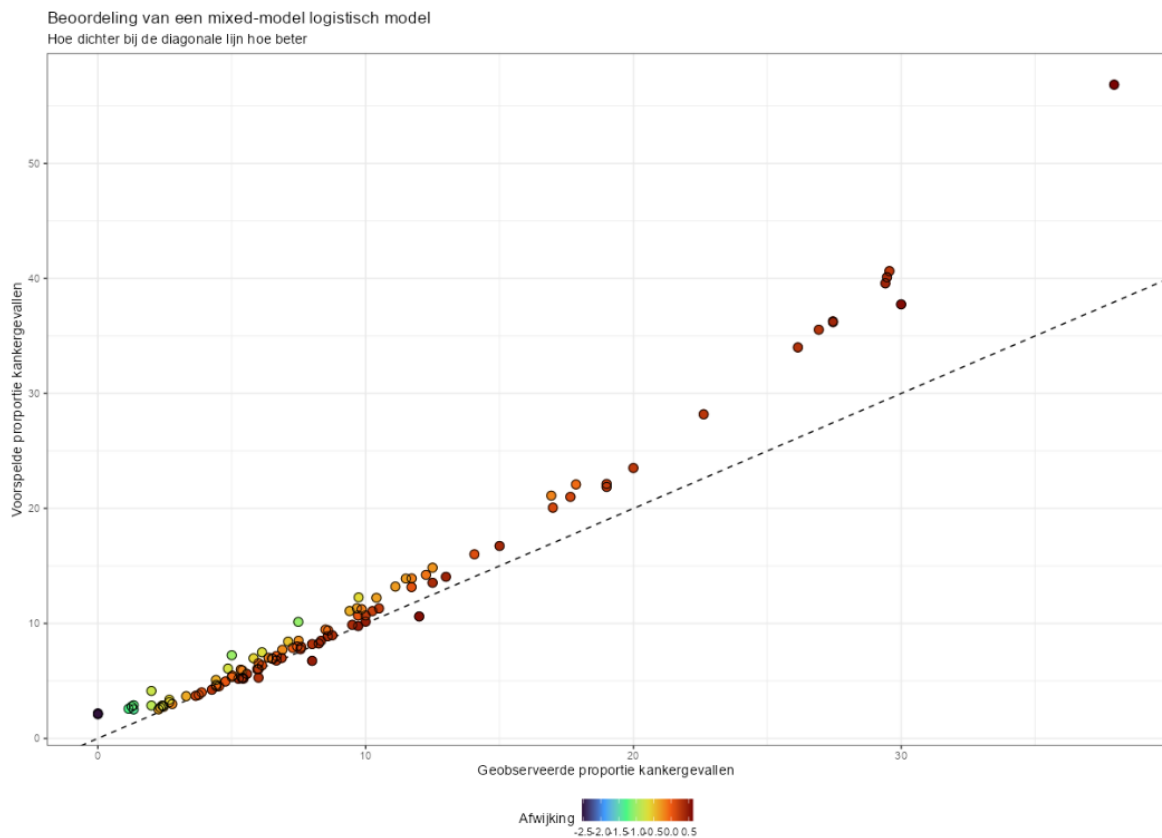
Figuur 110. De beoordeling van het GLMM model met binomiale verdeling en met splines. Dit model laat een vele sterkere correlatie zien tussen geobserveerde en voorspelde proporties kankergevallen, maar neigt sterk naar overfitting .
