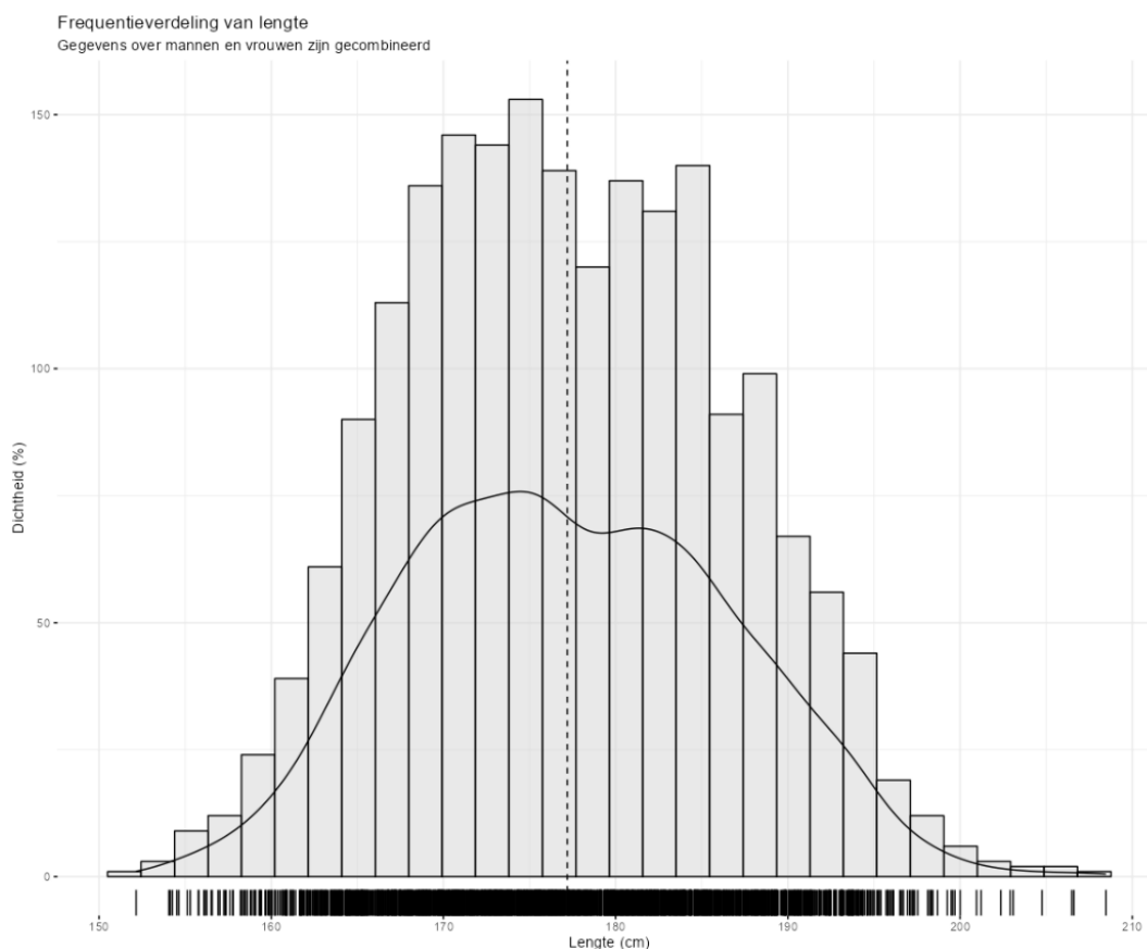
Figuur 12. De verdeling van lengte waarbij de gegevens van mannen en vrouwen zijn gecombineerd. De gegevens zijn gesimuleerd.
