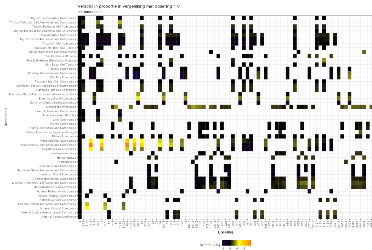
Figuur 65. Absolute verschil in proporties tussen de nuldosering en de andere doseringen per tumorsoort.
