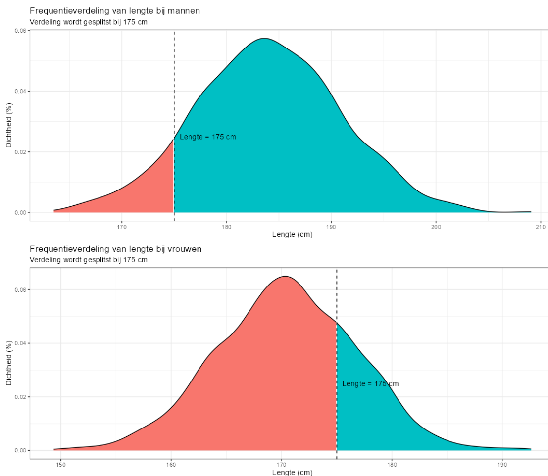
Figuur 16. De plek van 175 cm in de verdeling van Nederlandse mannen en van vrouwen.
