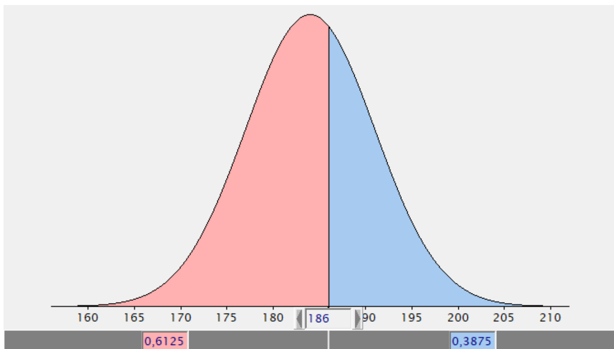
Figuur 6. De plek waar een lengte van 186 cm past in een verdeling van lengtes van Nederlandse mannen.
