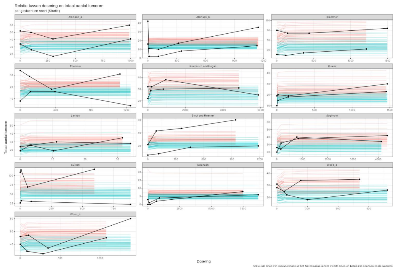
Figuur 152. Grafiek die relatie laat zien tussen dosering en aantal tumorgevallen, per geslacht en studie, op de originele schaal. De geobserveerde data (zwarte lijnen) lijken meer zeker dan de modelvoorspellingen aangeven.
