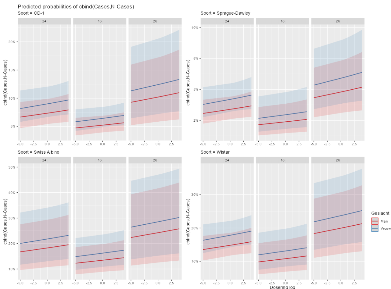
Figuur 108. De voorspellingen uit het GLMM model zoals weergegeven in Figuur 106 .
