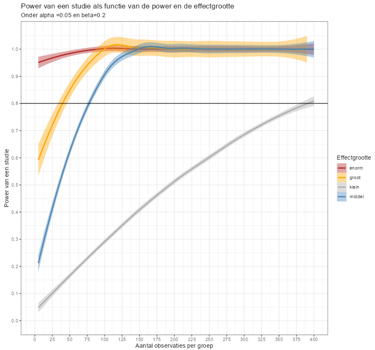
Figuur 35. Relatie tussen aantal observaties per groep, de effectgrootte tussen groepen en de kracht van een studie bij een \alpha waarde van 0.05 en een \beta waarde van 0.2.
