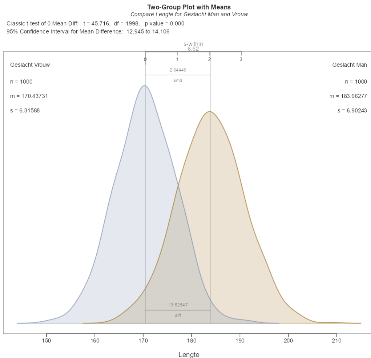
Figuur 24. De verdeling van lengtes voor mannen en vrouwen, met daarbij informatie over het gemiddelde (m), de standaard deviatie (s), het verschil (diff) en het gestandaardiseerde verschil (smd).
