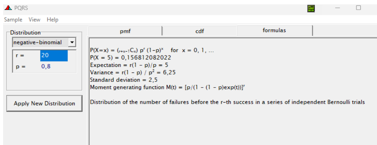
Figuur 130. Formules die bij de negatieve binomiale verdeling horen plus de uitkomsten bij r=20 en p=0.8 .
