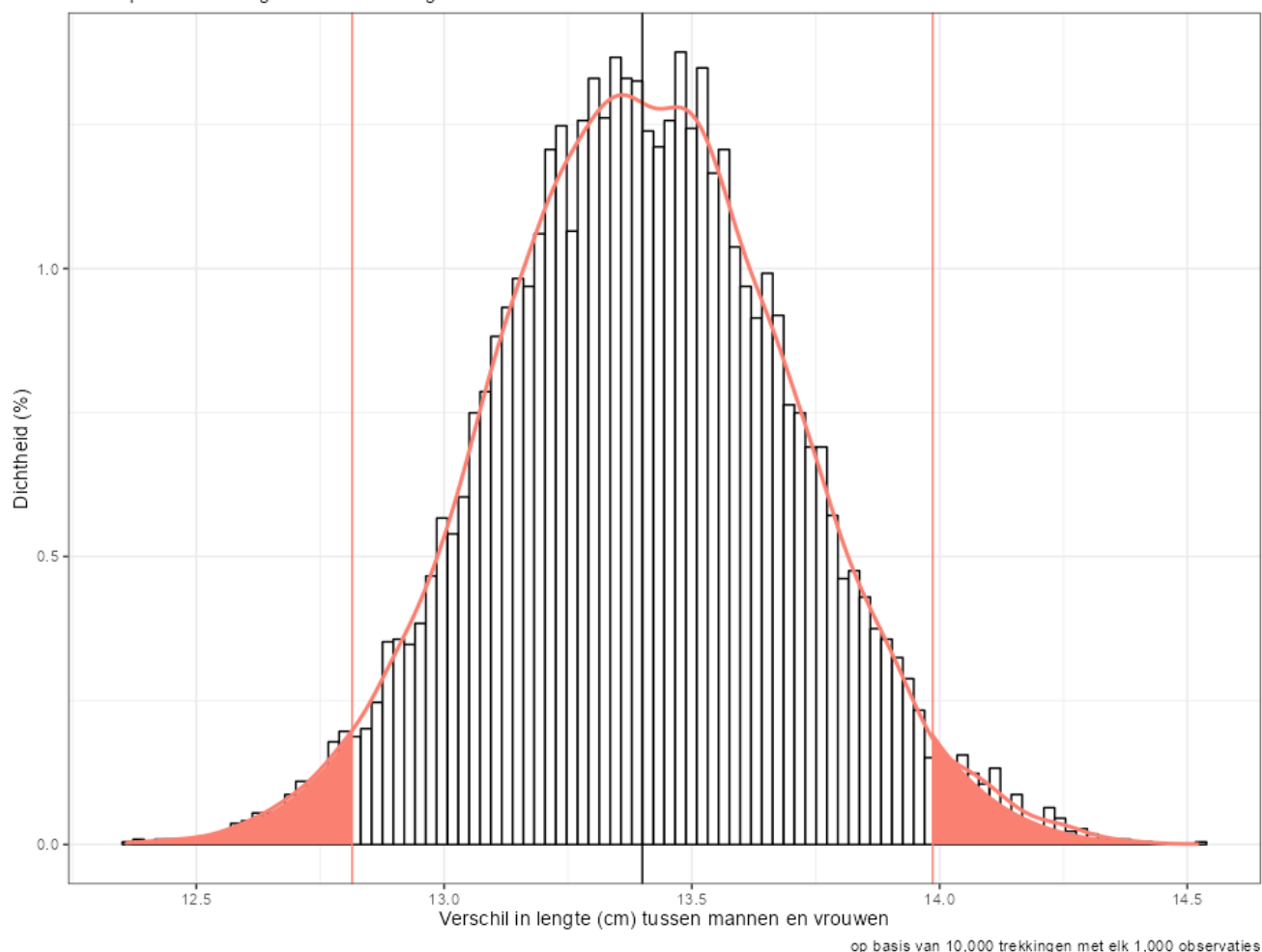
Figuur 27. De verdeling van gesimuleerde verschillen met in het midden de zwarte lijn die het gemiddelde verschil toont (13.4 cm). De rode lijnen zijn de 95% betrouwbaarheidsintervallen. We zien geen enkele keer de waarde 0.
