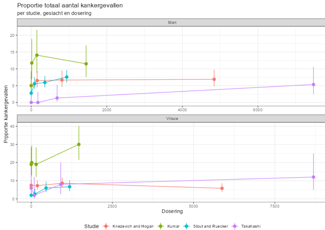
Figuur 174. Kans op kanker voor vier studies met onzekerheidsmarges.
