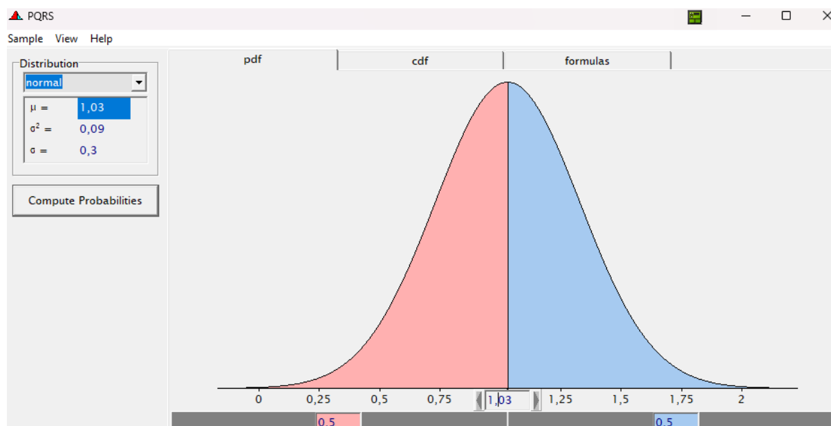
Figuur 136. Voorbeeld van een normaalverdeling met gemiddelde 1.03 en standaard deviatie 0.3 die zou kunnen gelden als prior voor de parameter Dosering .
