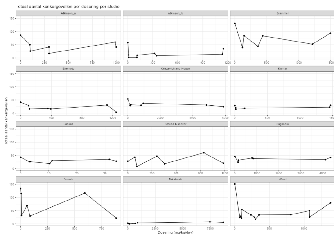
Figuur 67. Totaal aantal kankergevallen per dosering per studie.
