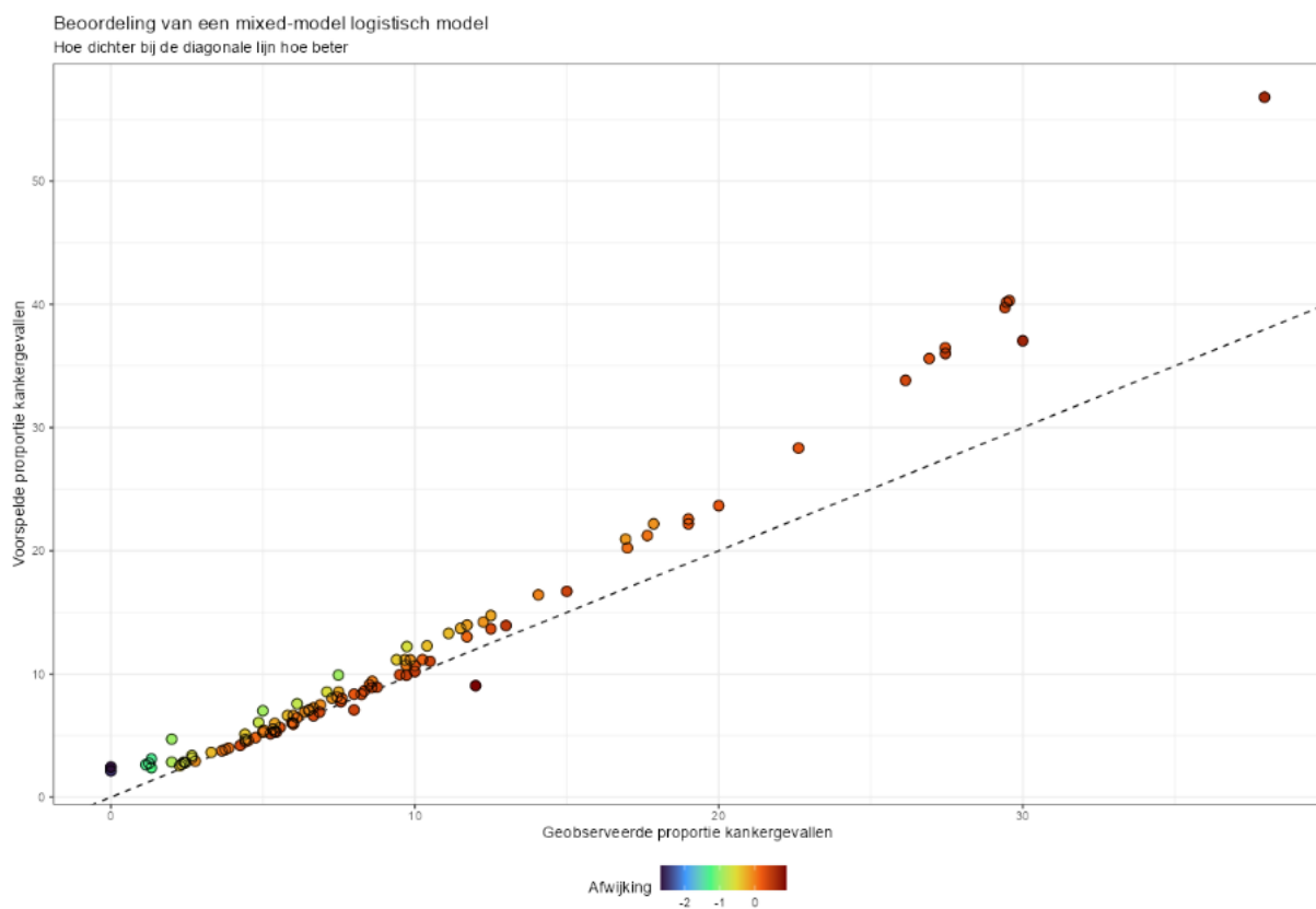
Figuur 114. De correlatie tussen geobserveerde en voorspelde proporties kankergevallen uit een GLMM model met interactie tussen dosering en geslacht.
