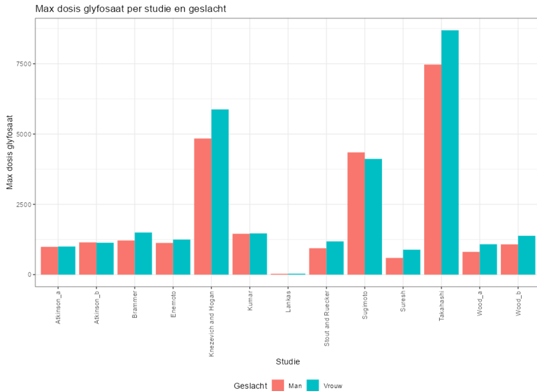
Figuur 172. Max dosis glyfosaat per studie en geslacht.
