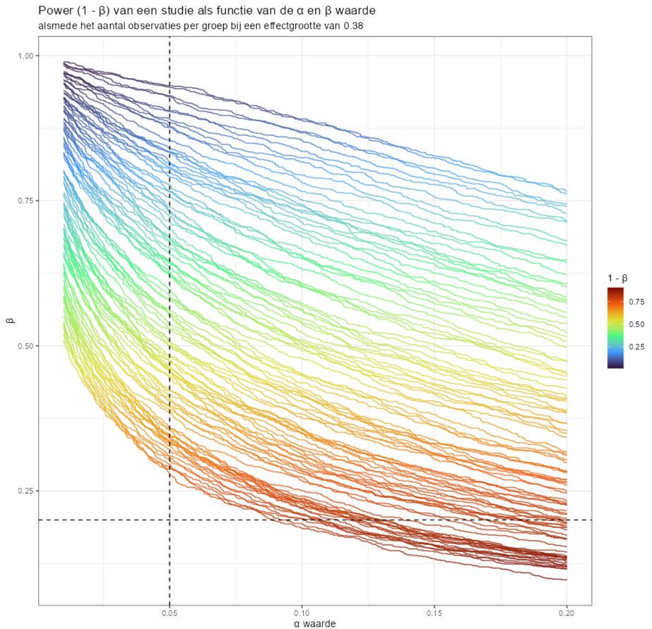
Figuur 39. De relatie tussen de \alpha en \beta waarde van een studie en de kracht om een effect te vinden.
