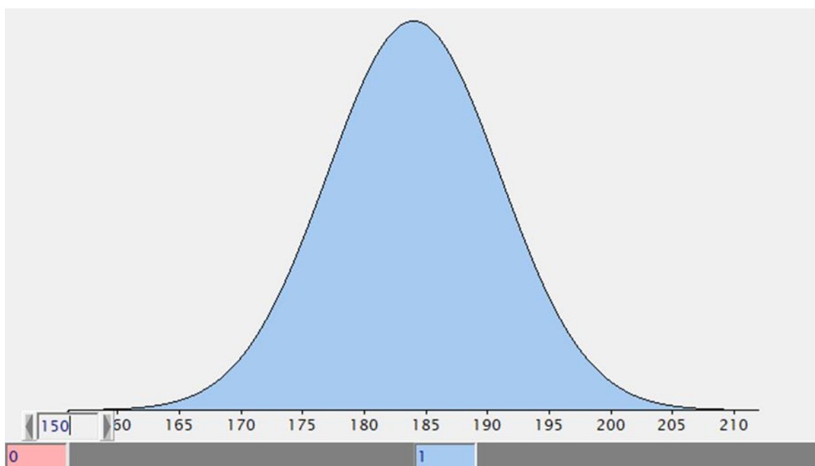
Figuur 10. De plek waar een lengte van 150 cm past in een normaalverdeling van lengtes van Nederlandse mannen.
