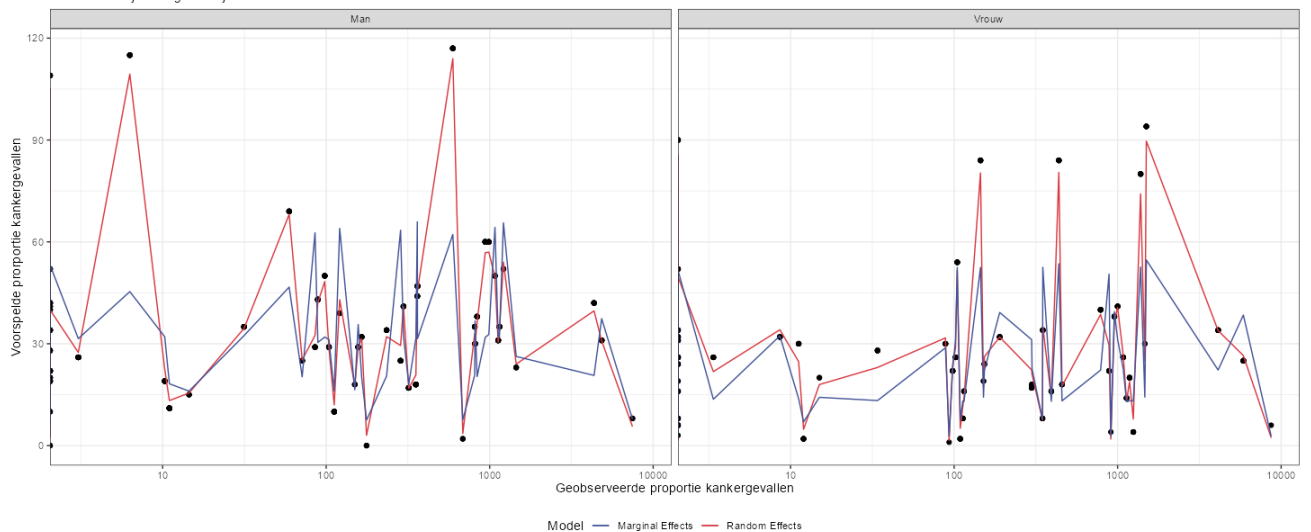
Beoordeling van een Mixed-Model met Poisson verdeling Hoe dichterbij de diagonale lijn hoe beter
