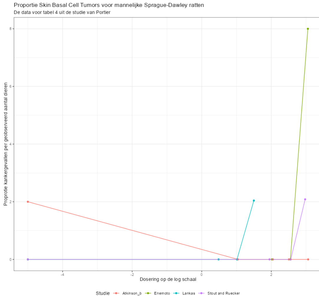
Figuur 121. Relatie tussen dosering en de proportie Skin Basal Cell Tumors voor mannelijke Sprague-Dawley ratten.
