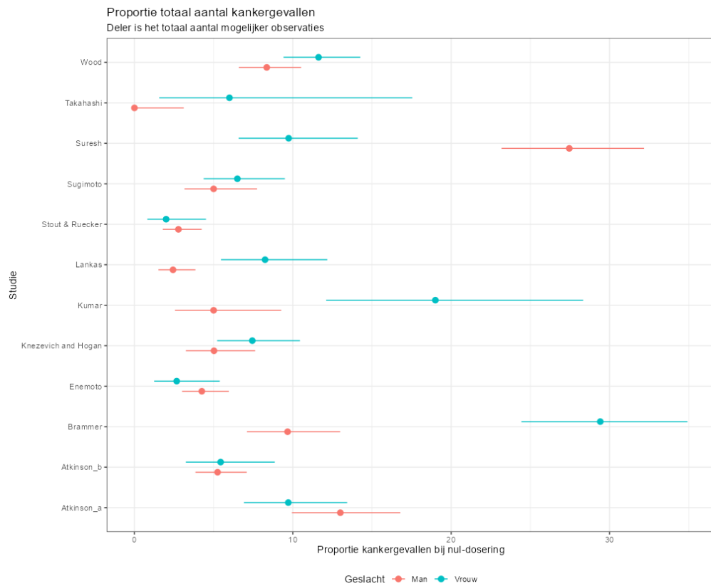
Figuur 103. Proportie kankergevallen bij nul-dosering waarbij de deler het totaal aantal mogelijke observaties is.
