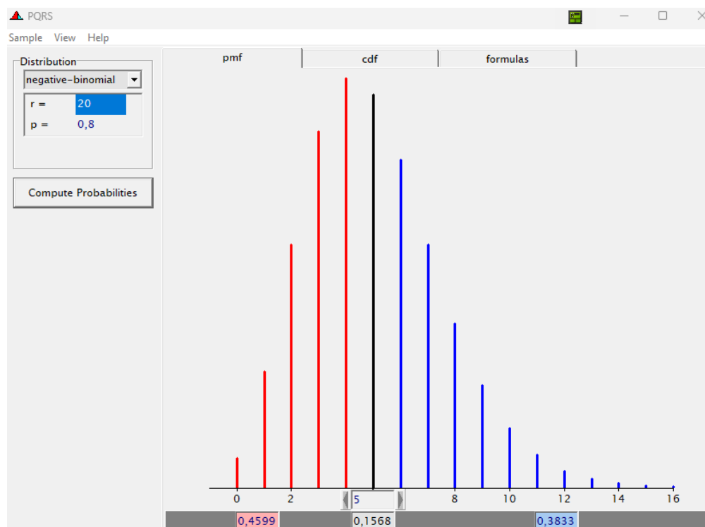
Figuur 129. Voorbeeld van een verdeling op basis van de negatieve binomiale verdeling.
