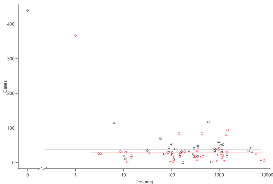
Figuur 82. Dose-response relatie op basis van alle data. Gekeken is naar het aantal gerapporteerde tumorgevallen, los van het aantal geïncludeerde dieren. Zoals te zien valt is het haast onmogelijk om een dose-response curve te maken.
