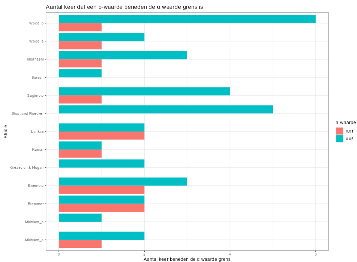
Figuur 77. Per studie het aantal toetsen dat onder een gespecificeerde grenswaarde viel. Dit zijn resultaten zoals door Portier gerapporteerd.
