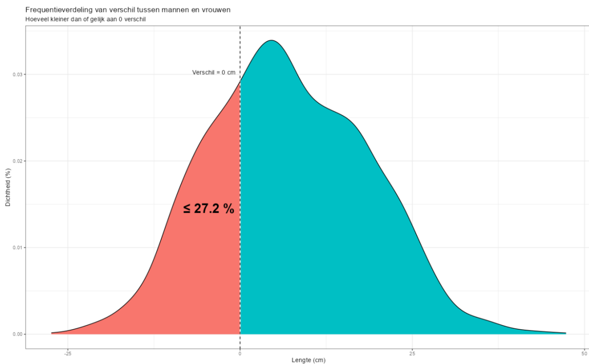
Figuur 19. De verdeling van verschillen. Ongeveer 27% van de waarden zijn negatief.
