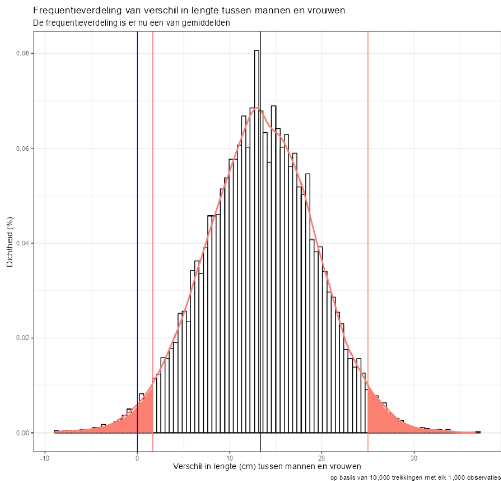
Figuur 28. De verdeling van verschillen wanneer de spreiding van beide groepen een factor 20 is van de originele spreiding. We zien nu voor het eerste de blauwe lijn van ‘geen verschil’ maar deze valt buiten de grenswaarde zodat we alsnog de nulhypothese van ‘geen verschil’ verwerpen.
