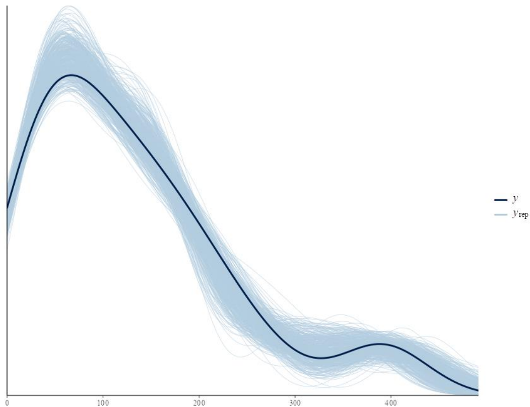
Figuur 161. Posterior verdeling ten opzichte van geobserveerde verdeling (donkere lijn).
