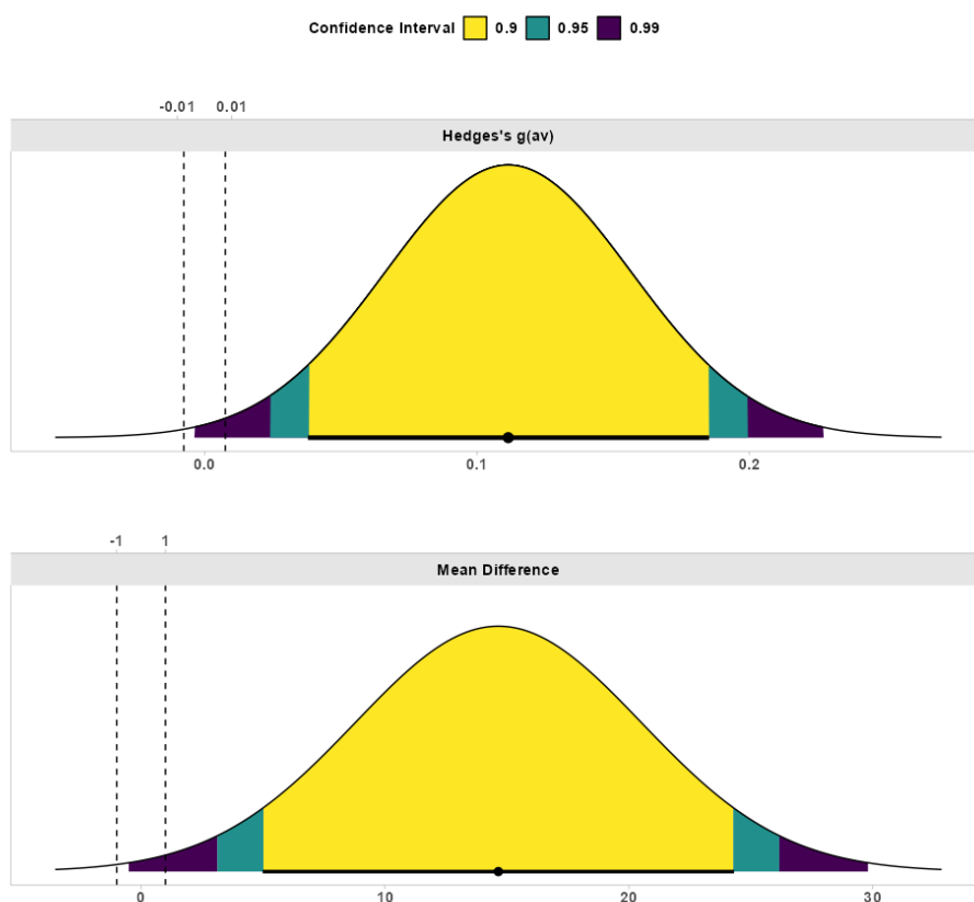
Figuur 47. Verschil tussen mannen en vrouwen in lengte waarbij de klinische grens op -1 én 1 is gezet. Het resultaat in de onderste grafiek laat zien dat het 99% betrouwbaarheidsinterval zowel de 1 als de 0 overschrijdt. Daarmee is het verschil tussen mannen en vrouwen niet statistisch significant én niet statistisch equivalent. We kunnen dus niet zomaar de nulhypothese van 'geen verschil' aannemen ook al is het verschil statistisch significant.
