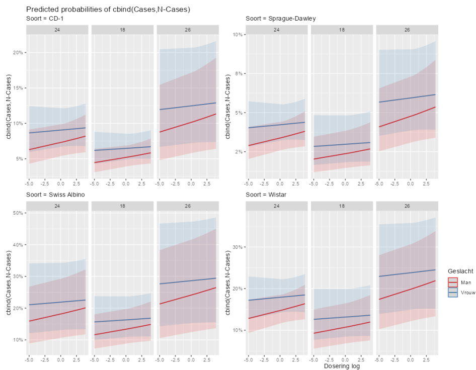
Figuur 113. Voorspelde proporties aan kanker voor een GLMM model met binomiale verdeling en een interactie tussen dosering en geslacht.
