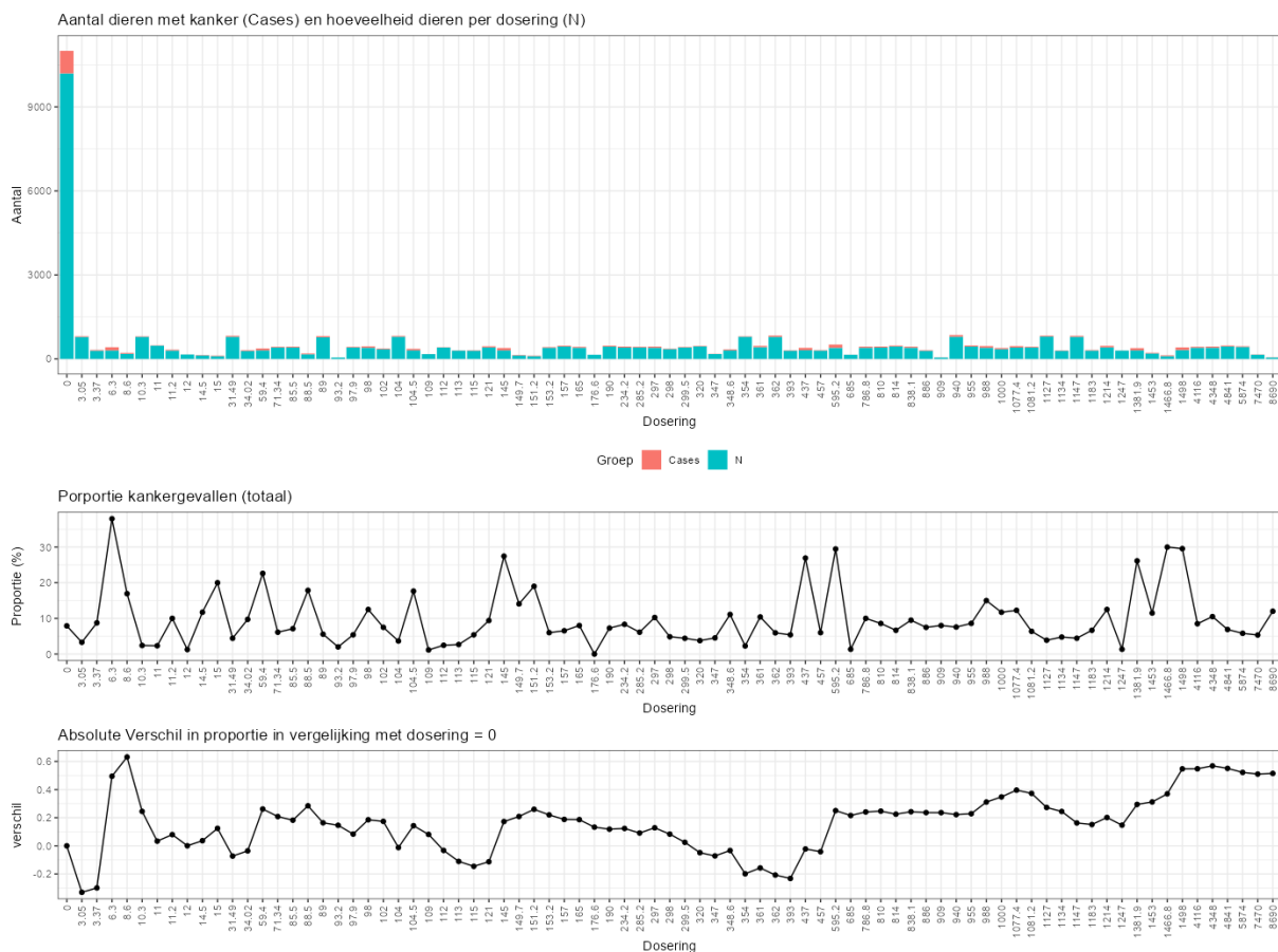
Figuur 62. Aantal dieren met kanker en hoeveelheid dieren per dosis (bovenste figuur);proportie kankergevallen per dosis (middelste figuur); én absolute verschil in proporties tussen de nuldosering en de andere doseringen (onderste figuur).
