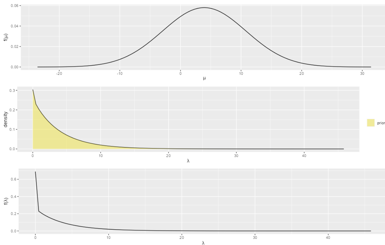
Figuur 154. Drie verdelingen op basis van de geobserveerde data. Van boven naar beneden: de normaalverdeling, de gamma verdeling en de gamma-poisson verdeling. De gamma-poisson heet ook wel de negatieve binomiale verdeling en die hebben we al veelvuldig voorbij zien komen.
