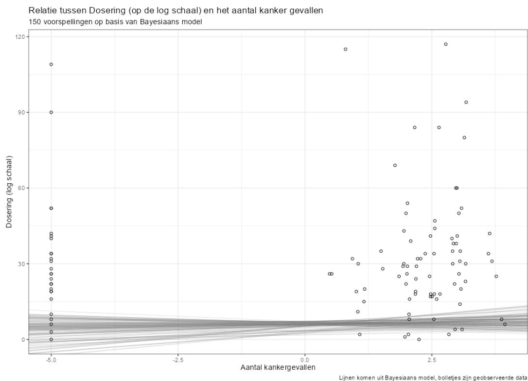
Figuur 144. Voorspellingen (lijnen) en geobserveerde waarden in de relatie tussen dosering en het aantal kanker gevallen. In dit voorbeeld neem ik alleen de marginale (gemiddelde) parameter waarden mee. Ik neem in dit voorbeeld niet de correctie voor studie mee.
