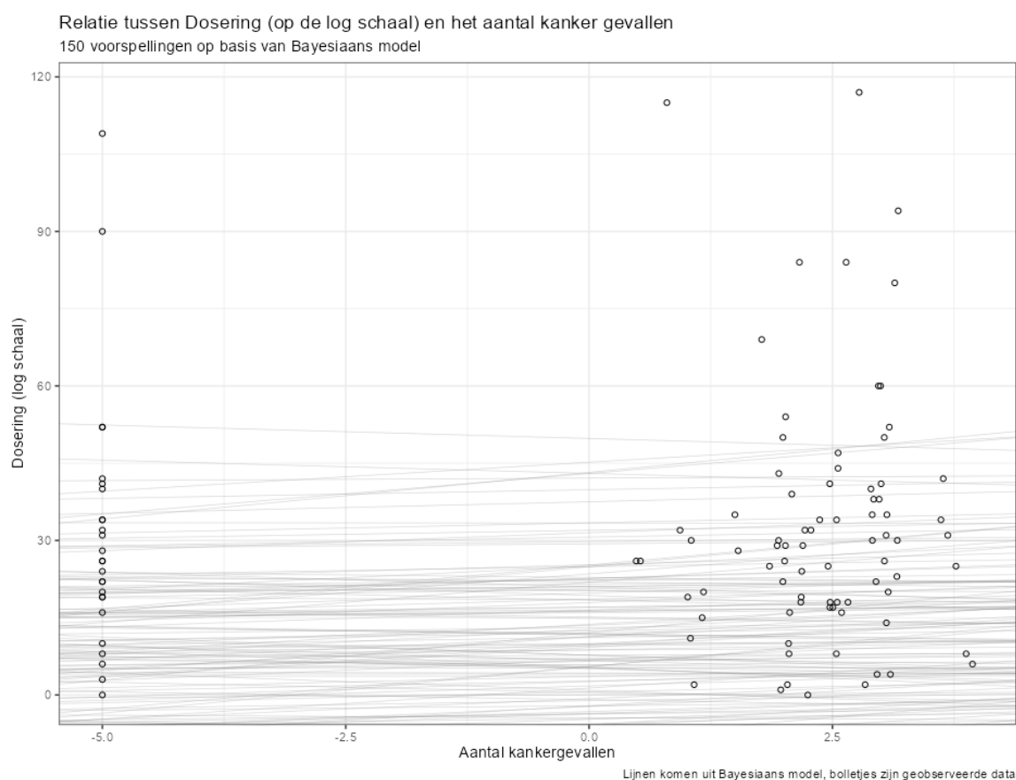
Figuur 145. Voorspellingen en geobserveerde waarden waarbij de correctie voor studie wel wordt meegenomen. Duidelijk zichtbaar, in vergelijking met Figuur 144 , is de toename in spreiding vanuit de schattingen.
