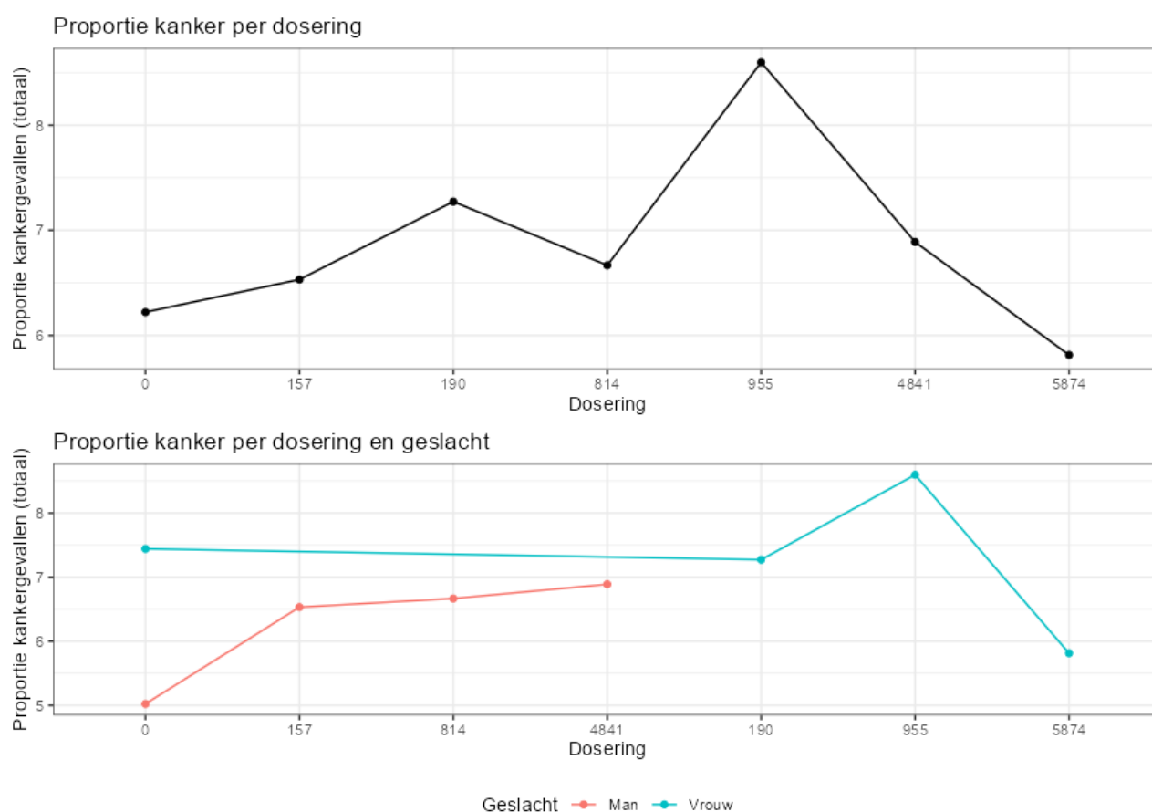
Figuur 56. Proportie kanker per dosering, en per dosering én geslacht.
