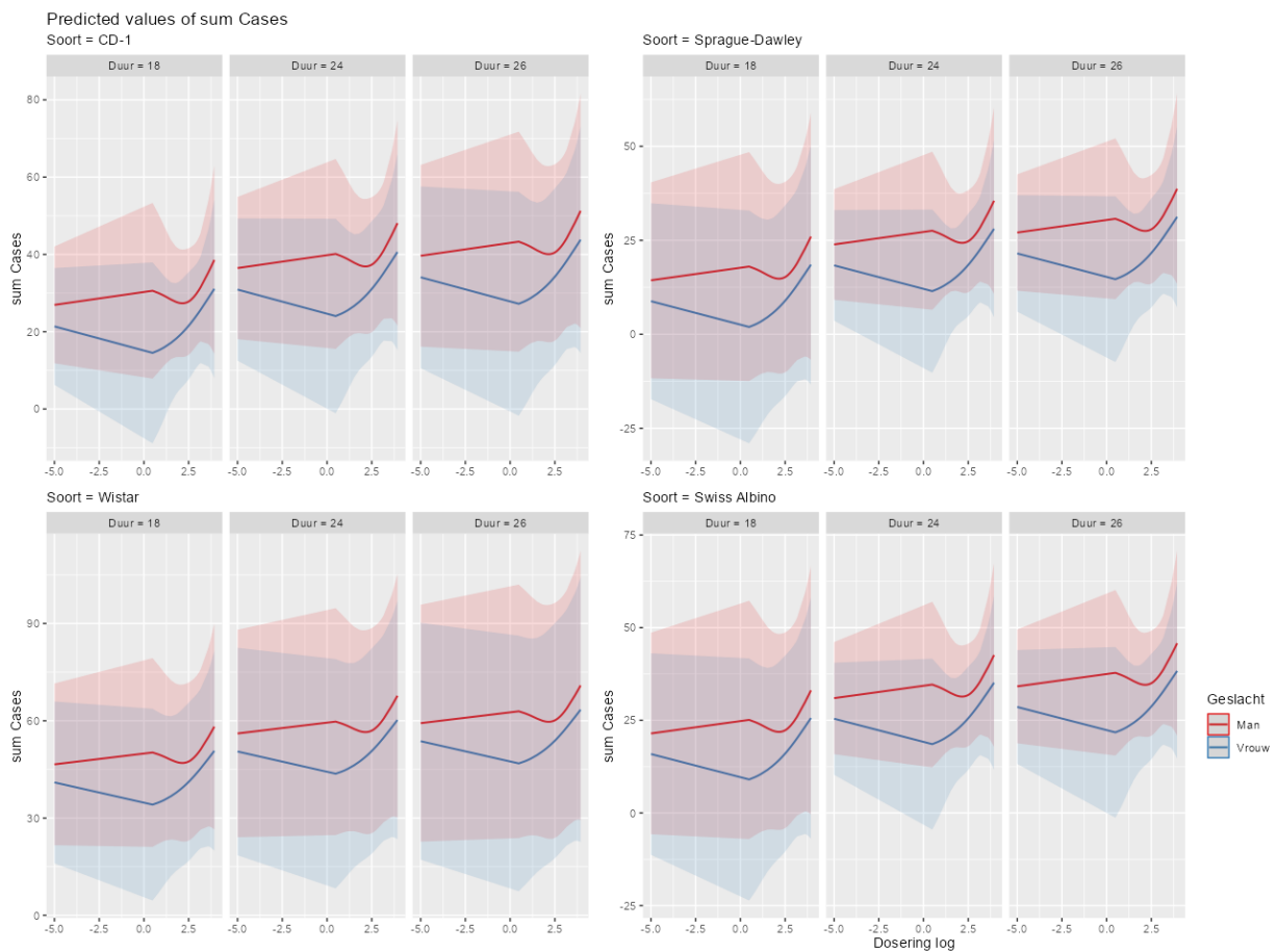
Figuur 95. Een LMM met natural splines die gek gedrag laat zien. Dit is geen behulpzaam model.
