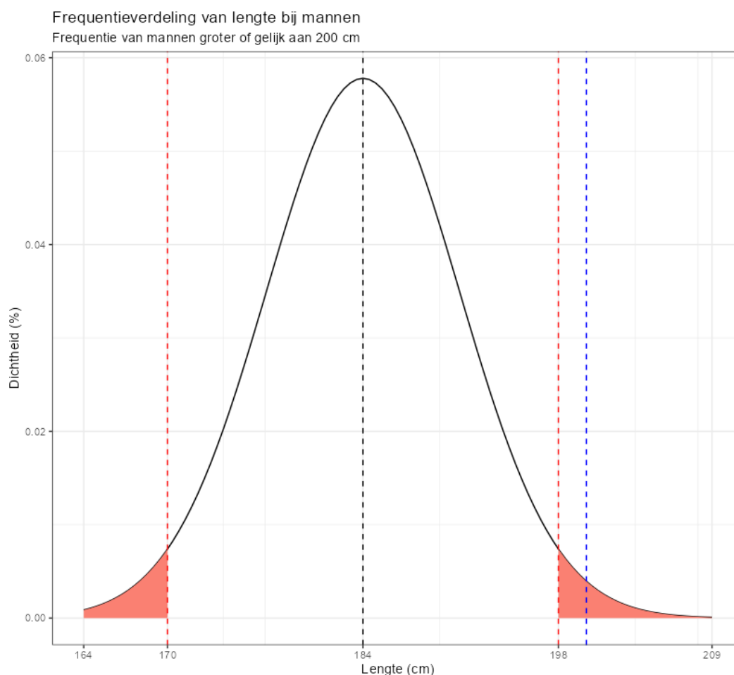
Figuur 21. De 2,5% grenswaardes links en rechts van het gemiddelde afgevinkt met een rode stippellijn. De zwarte stippellijn is het gemiddelde en de blauwe stippellijn laat zien waar de 200 cm valt.
