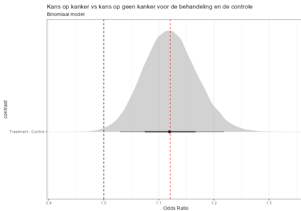
Figuur 164. De odds-ratio voor het verschil tussen de controlegroep en de behandelgroep.
