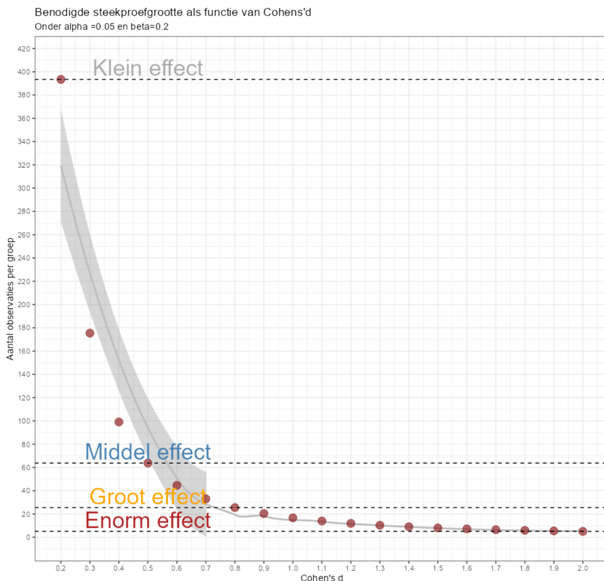
Figuur 36. Relatie tussen effectgrootte (Cohen's d) en het aantal observaties per groep. De stippellijnen laten zien wat de minimale grootte per groep moet zijn onder een \alpha van 0.05 en een \beta van 0.2.
