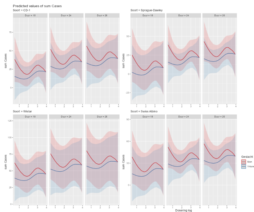
Figuur 99. Non-lineaire relatie op basis van natural splines vanuit een model zonder nul-dosering. In dit model valt heel duidelijk te zien dat de relatie tussen dosering en opgeteld aantal kankergevallen gekke patronen begint te vertonen. Deze patronen zijn niet echt, maar eerder het gevolg van grote onderlinge variatie gecombineerd met een model wat aan overfitting doet.
