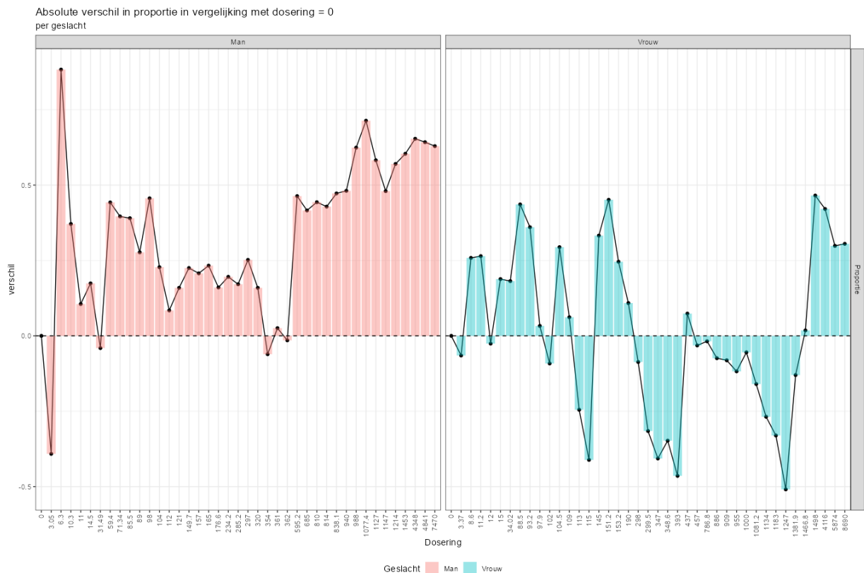
Figuur 63. Absolute verschil in proporties tussen de nuldosering en de andere doseringen per geslacht.
