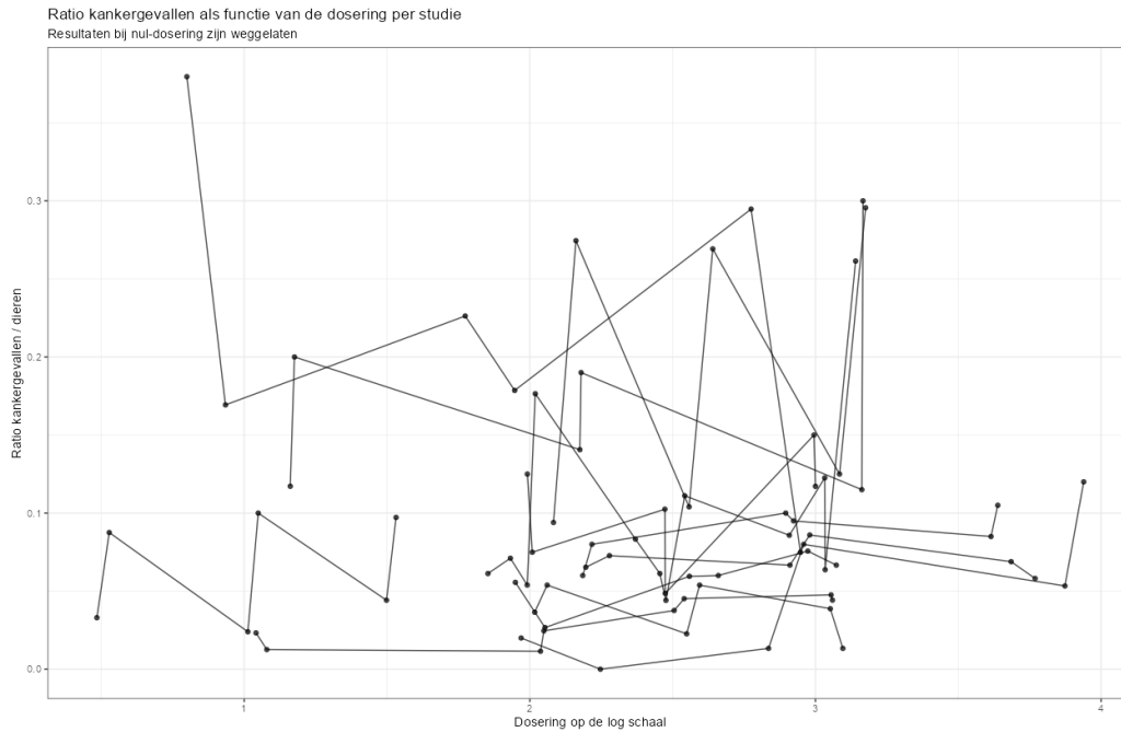
Figuur 86. Ratio kankergevallen als functie van de dosering per studie. Elke lijn is een studie. Deze keer is de nul-dosering weggelaten.
