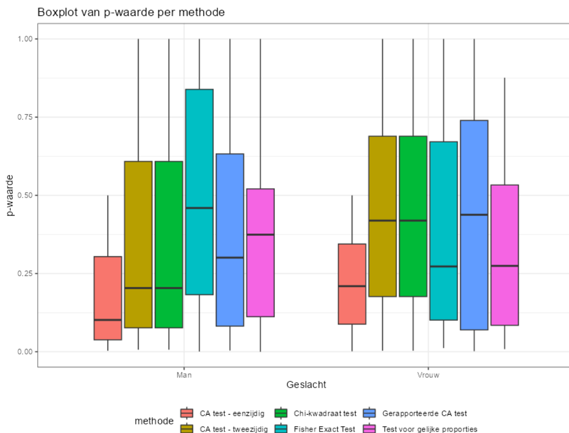
Figuur 70. Boxplot die de verdeling van p-waardes laat zien per methode én geslacht.
