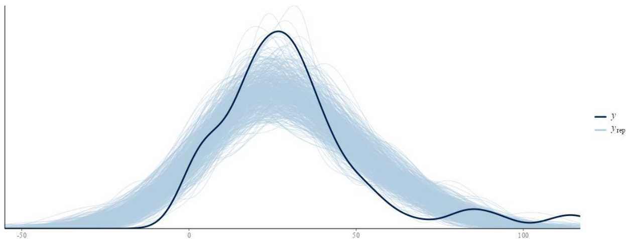
Figuur 139. Posterior check van het model. De donkere lijn is de geobserveerde waarde – de dunne lijnen zijn trekken uit de verdelingen afkomstig van het model.
