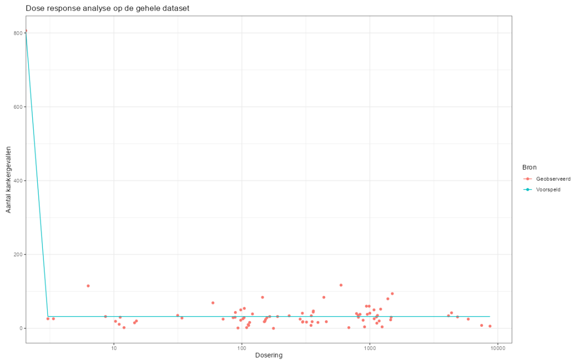
Figuur 60. Dose-response curve waarbij de dosering wordt afgezet tegenover het aantal kankergevallen. De blauwe lijn is de lijn afkomstig van een wiskundig model met als data de rode bolletjes: dit zijn alle observaties.
