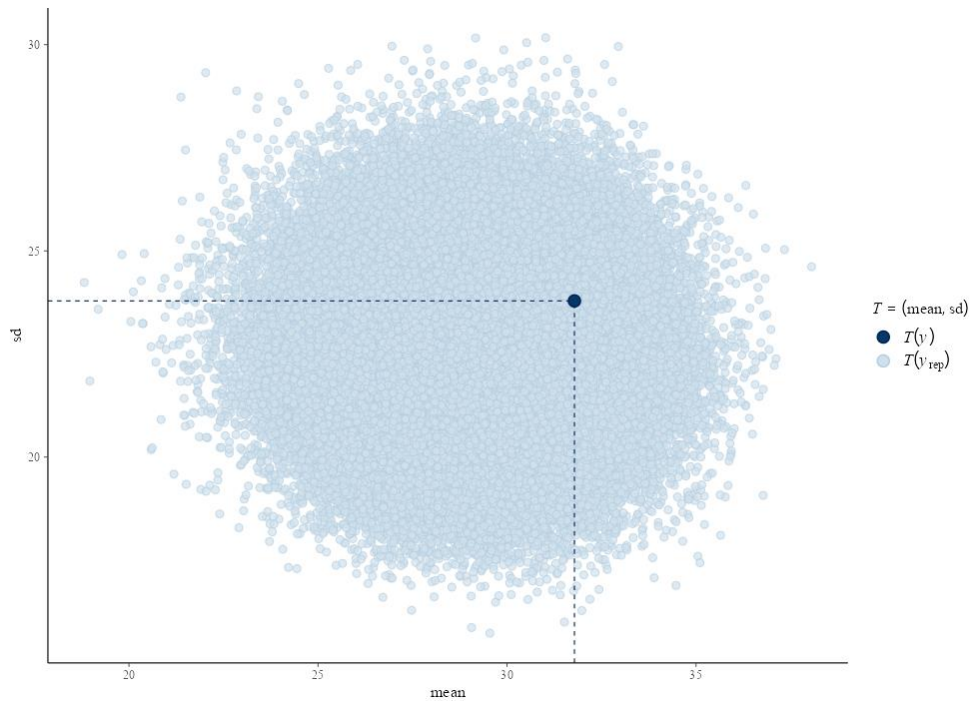
Figuur 141. Posterior check van het model waarbij zichtbaar wordt waar de afwijking tussen observatie en modelvoorspelling het grootst is.
