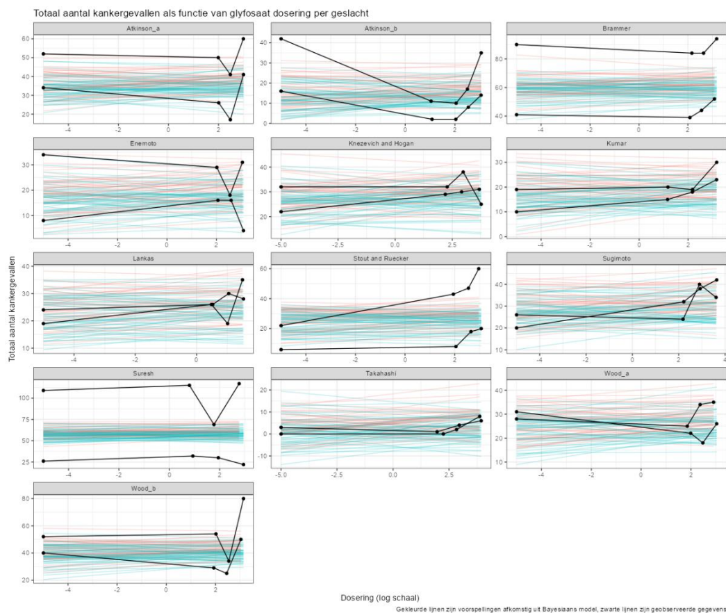
Figuur 147. Relatie tussen dosering en aantal kanker gevallen, per studie en per geslacht waarbij de gekleurde lijnen de voorspellingen zijn per geslacht en de zwarte lijnen en bolletjes de geobserveerde waarden zijn. Het gaat hier om totale kanker gevallen per dosering per geslacht en per studie.
