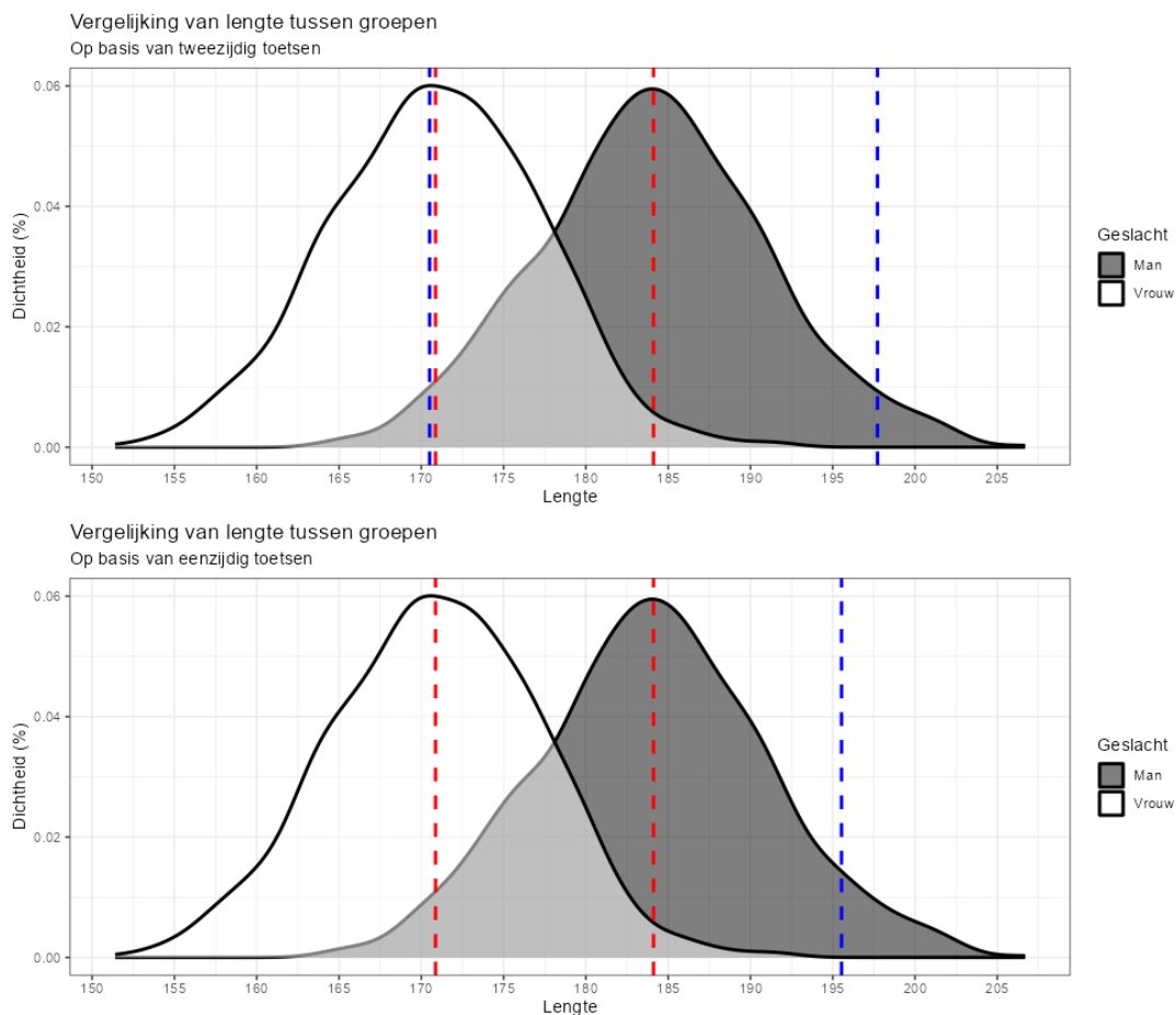
Figuur 44. Grenswaarde (blauwe stippellijn) als functie van tweezijdig en eenzijdig toetsen.
