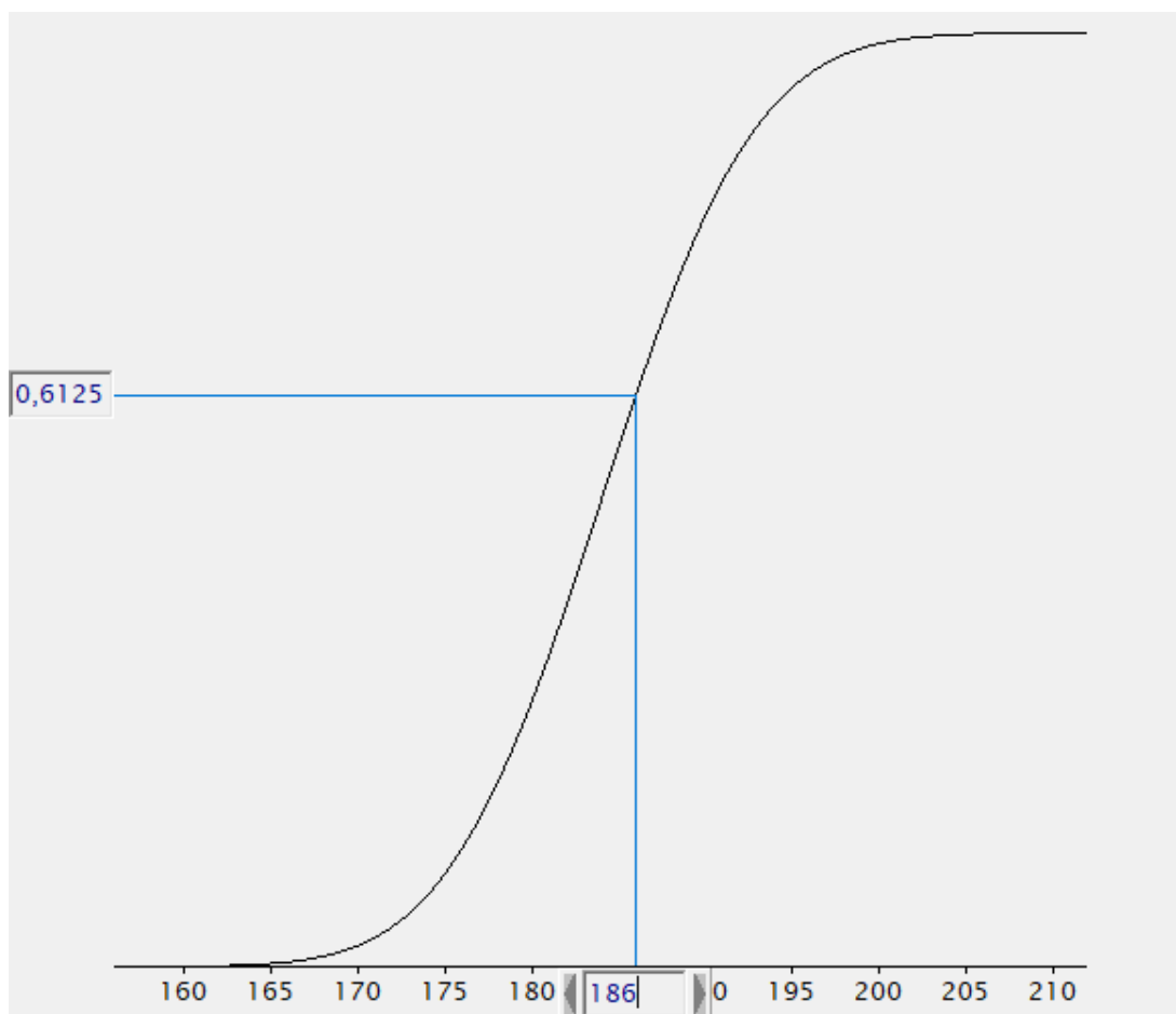
Figuur 7. De cumulatieve kansverdeling bij een gemiddelde van 184 cm met 7 cm standaarddeviatie.
