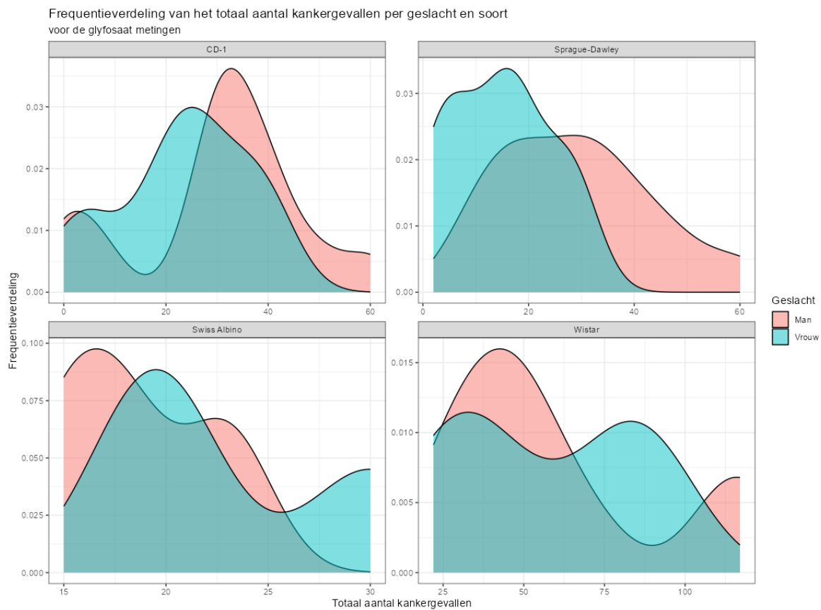
Figuur 159. Verdeling van het aantal kankergevallen per geslacht en soort over de glyfosaatverdelingen heen.
