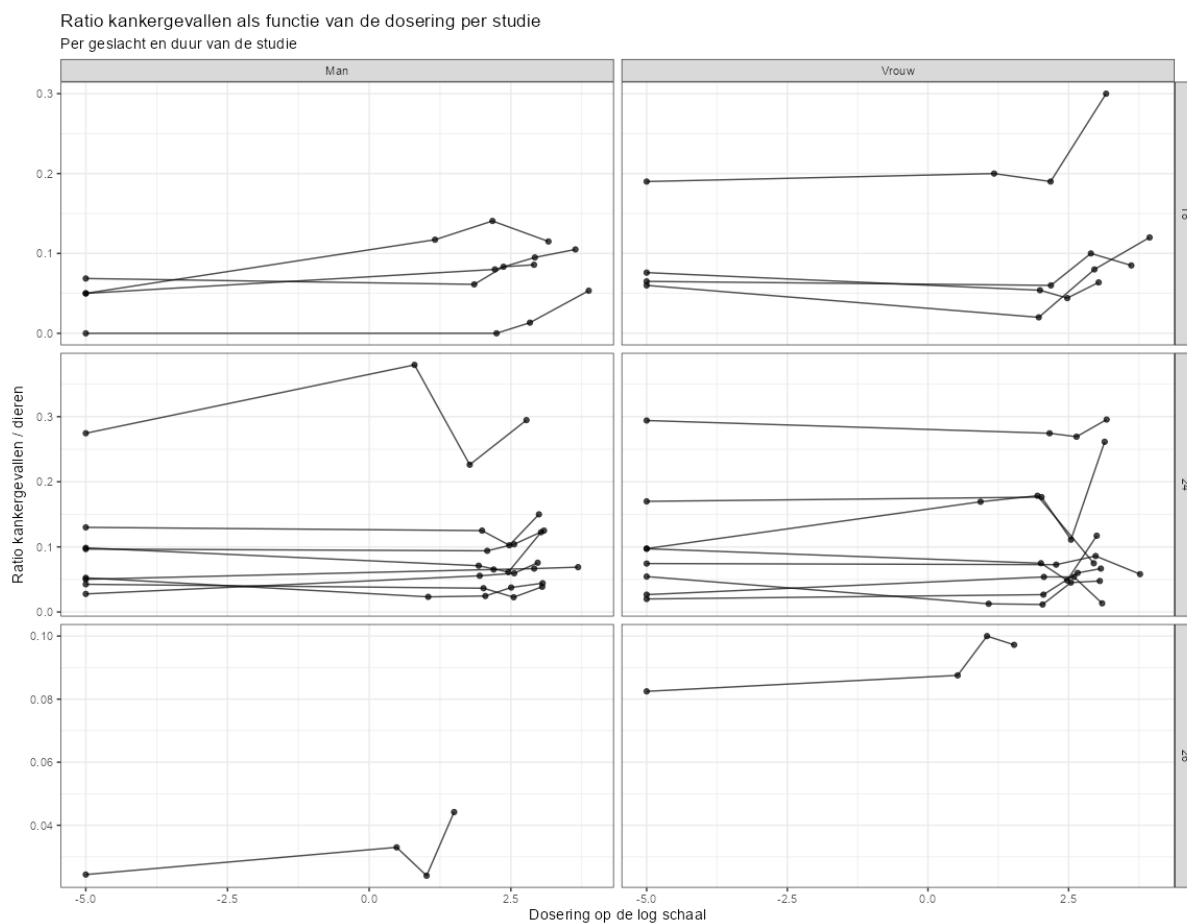
Figuur 84. Dose-response curve met op de x-as de dosering op de log schaal. Elke lijn is een studie. Op de Y-as is de ratio van het aantal kankergevallen per het aantal dieren zoals geïncludeerd per dosering. Een verder onderverdeling is gemaakt per geslacht (kolom) en de duur van de studie (rijen).
