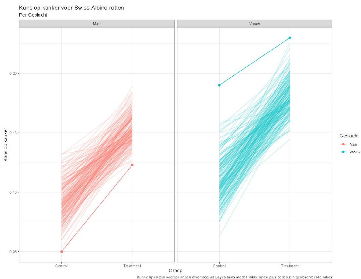
Figuur 170. De kans op kanker voor mannelijke en vrouwelijke Swiss-Albino ratten in de controlegroep en de behandelgroep. Het model wijkt af met een haast vaste constante wat een gevolg is van het type model.
