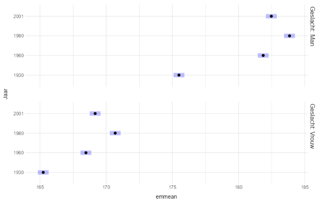
Figuur 54. Gemiddelde waarde en 95% betrouwbaarheidsinterval.
