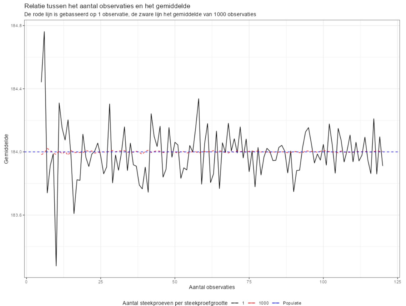
Figuur 31. Relatie tussen de schatting van het gemiddelde en de steekproefgrootte. De blauwe lijn is het theoretisch gemiddelde (184 cm). De zwarte en rode lijn zijn schattingen gebaseerd op 1 steekproef per steekproefgrootte en het gemiddelde van 1000 steekproeven, respectievelijk.
