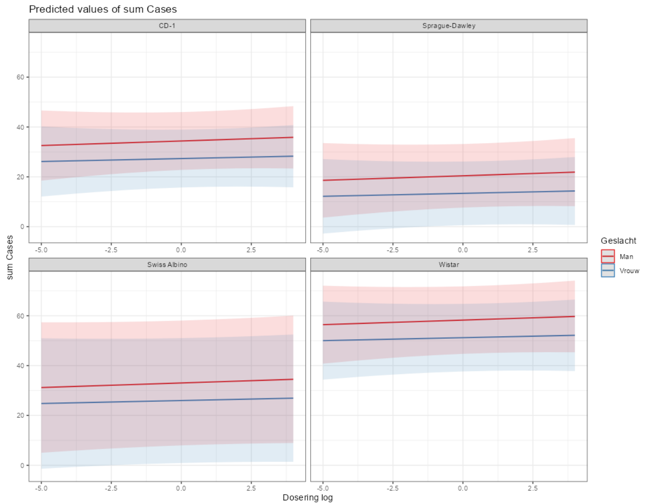
Figuur 91. Voorspellingen afkomstig van een LMM model met als y-variabele het opgeteld aantal kankergevallen ( sum Cases ). De lijn laat de voorspelde waarde zien als functie van de dosering (log schaal), geslacht en soort.
