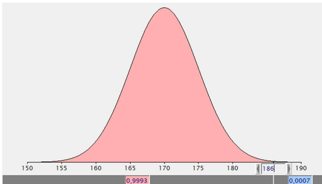
Figuur 11. De plek waar 186 cm past in een normaalverdeling van lengte van Nederlandse mannen met een gemiddelde van 170 cm en een standaard deviatie van 5 cm.
