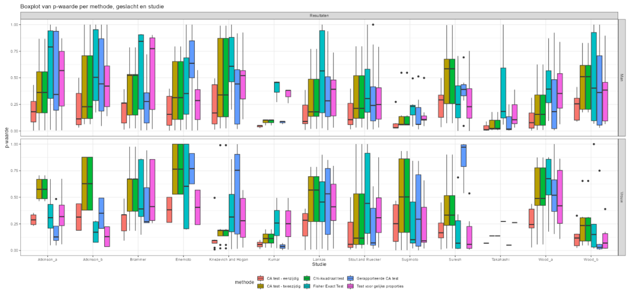
Figuur 71. Boxplot die de verdeling van p-waardes laat zien per methode, geslacht én studie.
