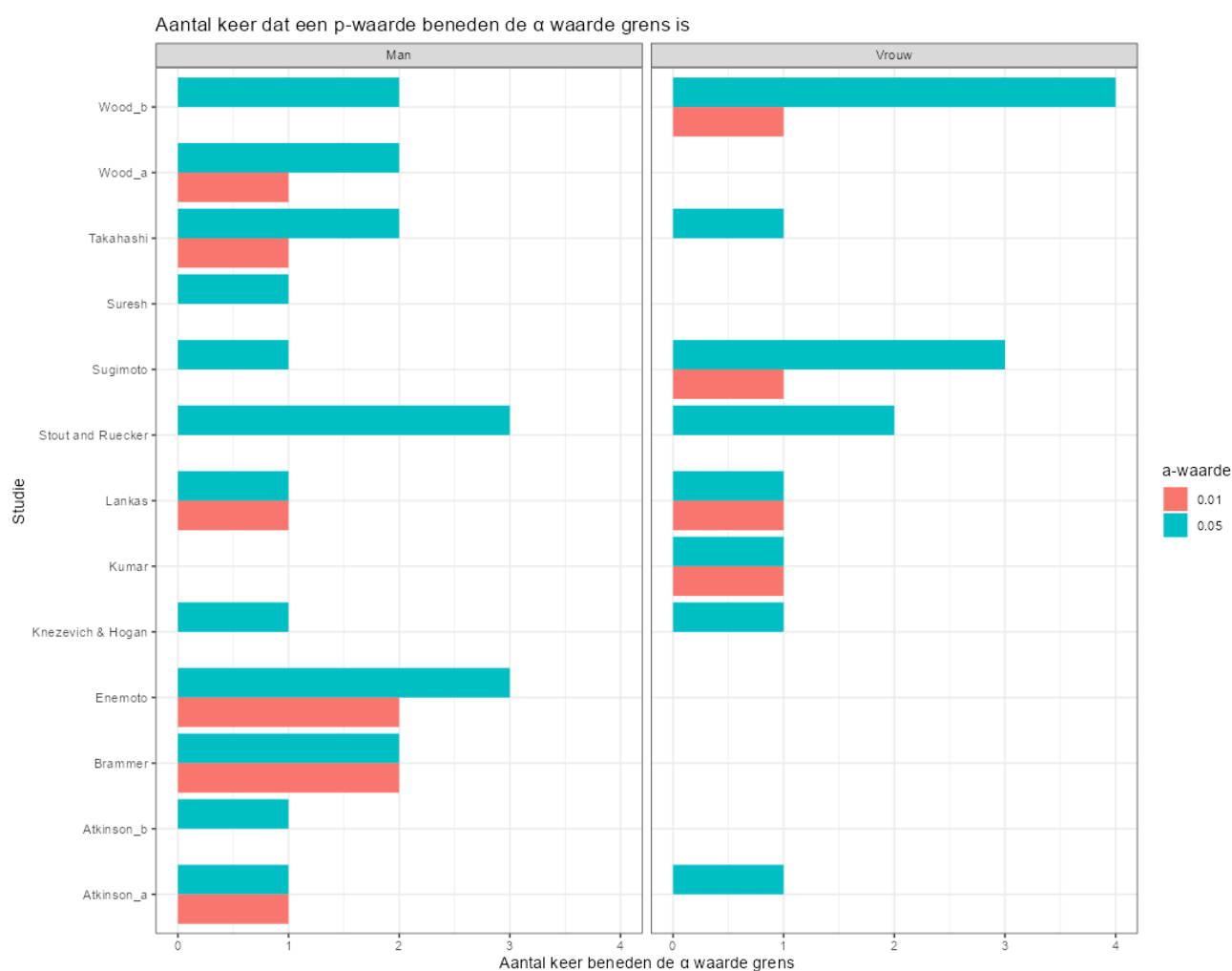
Figuur 78. Per studie en geslacht het aantal toetsen dat onder een gespecificeerde grenswaarde viel. Dit zijn resultaten zoals door Portier gerapporteerd.
