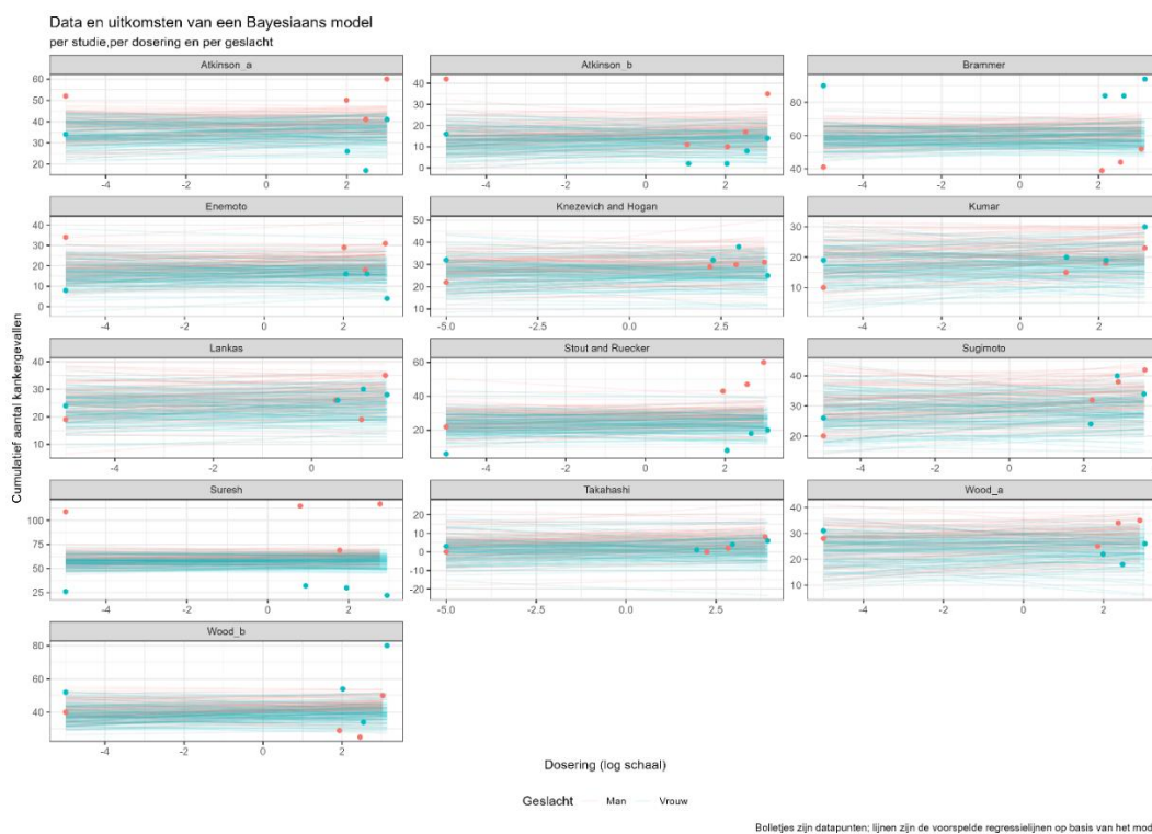
Figuur 143. Voorspellingen (lijnen) en geobserveerde waarden in de relatie tussen dosering en het aantal kankergevallen.
