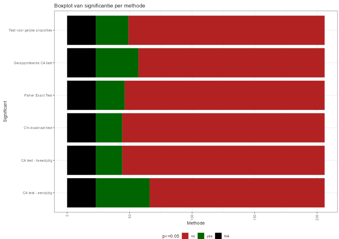
Figuur 72. Boxplot die per methode het aantal significante resultaten laat zien voor p \leq 0.05 . Daarmee is het een visuele representatie van Tabel 18. De eenzijdige CA test zoals door mij uitgevoerd laat het grootste aantal significante resultaten zien. Daarna komen de resultaten van Portier: het aantal ligt tussen de eenzijdige en tweezijdige CA test.
