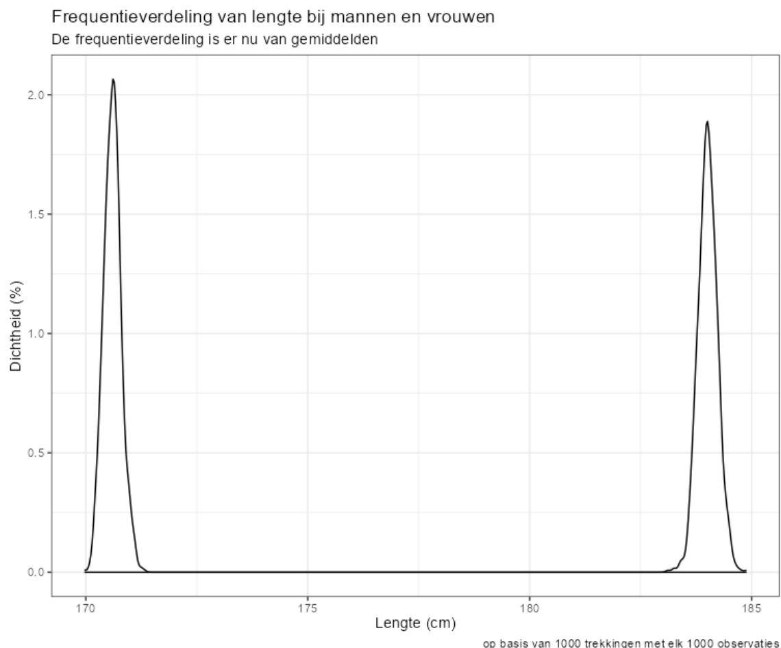
Figuur 25. De verdeling van gemiddeldes voor mannen en vrouwen. Het valt duidelijk te zien dat er tussen die gemiddeldes geen observaties zijn. Er is daadwerkelijk een kloof tussen twee torens.
