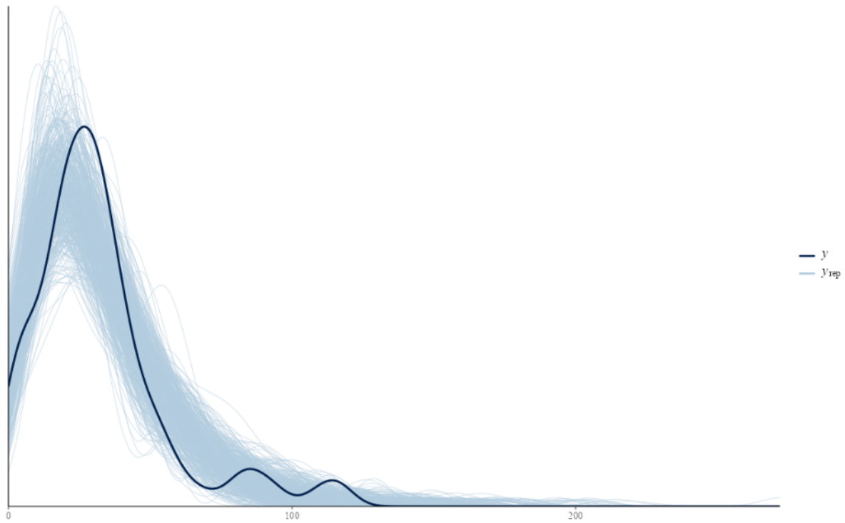
Figuur 150. De verdeling van de posterior voor een leeg hurdle model (lichte lijnen), en de verdeling van de geobserveerde tumorgevallen (donkere lijn).
