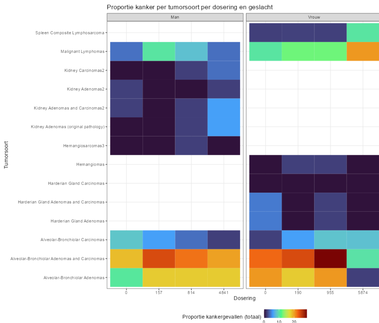
Figuur 57. Proportie kanker zoals verkregen vanuit Figuur 55 .
