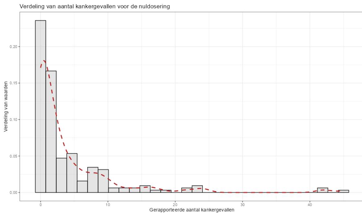
Figuur 153. Verdeling van het aantal kankergevallen bij de nul-dosering.
