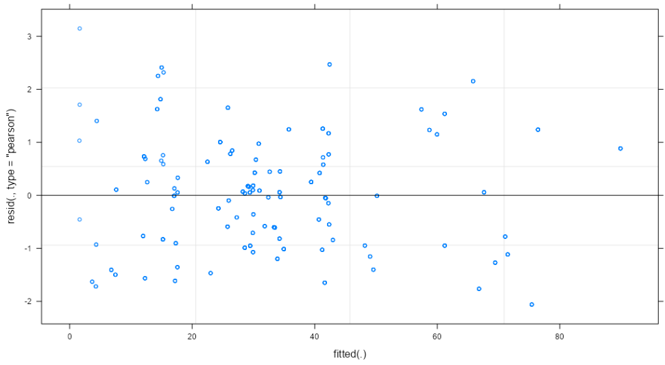
Figuur 131. Relatie tussen restwaarden van het model en het aantal kankergevallen.
