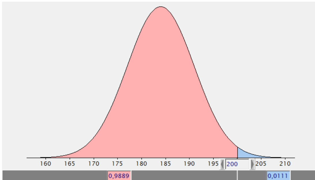
Figuur 8. De plek waar een lengte van 200 cm past in een normaalverdeling van lengtes van Nederlandse mannen.
