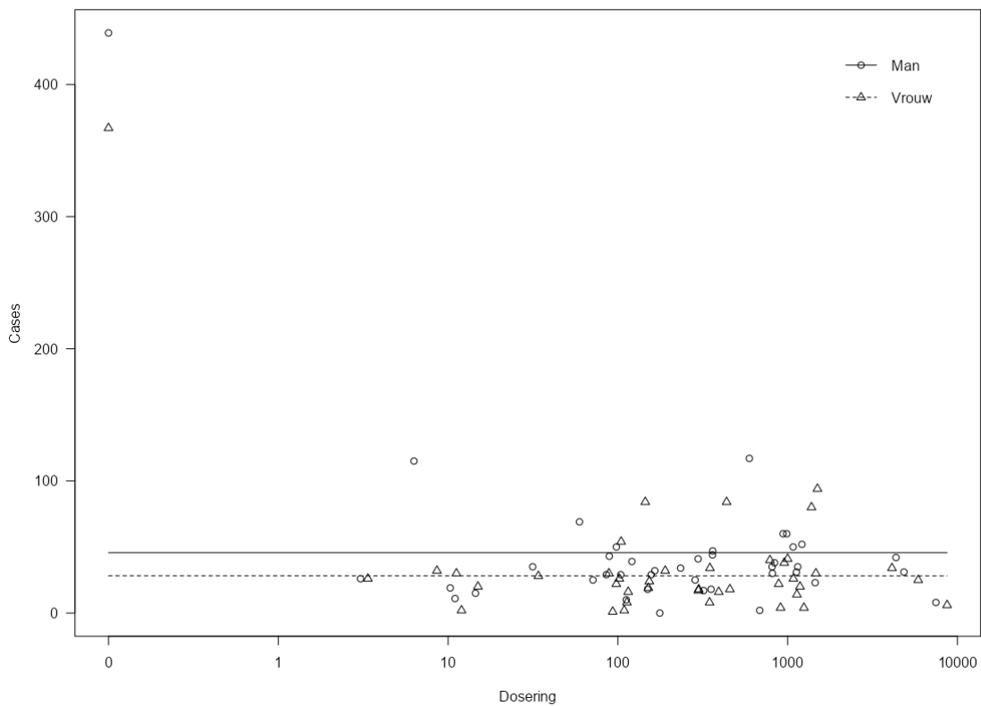
Figuur 61. Dose response per geslacht – exercitie is gelijk aan Figuur 60 .
