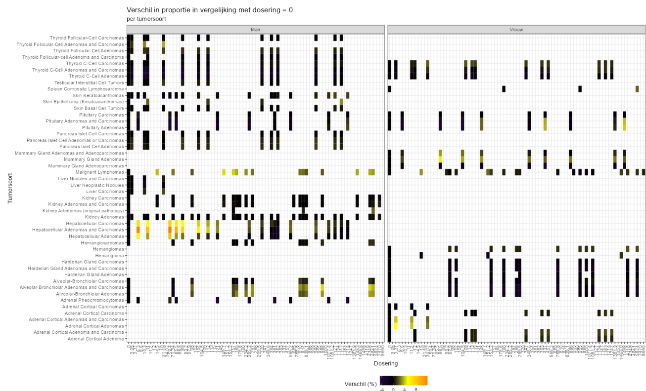
Figuur 66. Absolute verschil in proporties tussen de nul-dosering en de andere doseringen per tumorsoort en per geslacht.
