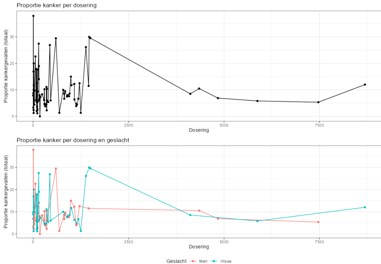
Figuur 59. Proportie kanker per dosering én proportie kanker per dosering en geslacht. Duidelijk te zien dat het gros van de studies data heeft verzameld tot ongeveer 2000 mg/kg/dag. De lineaire schaal is waarschijnlijk niet de beste schaal om mee te meten.
