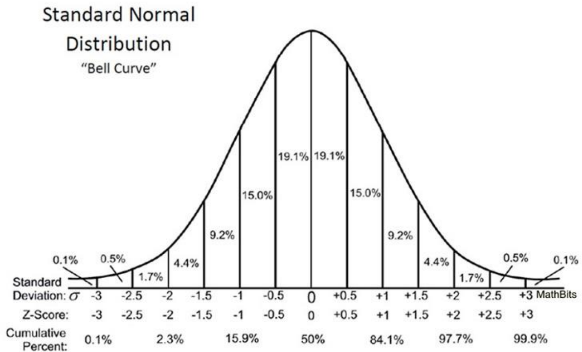
Figuur 5. Theoretische kansverdeling van de normaalverdeling met een gemiddelde 0 en standaard deviatie 1. Onderaan staan de cumulatieve percentages.
