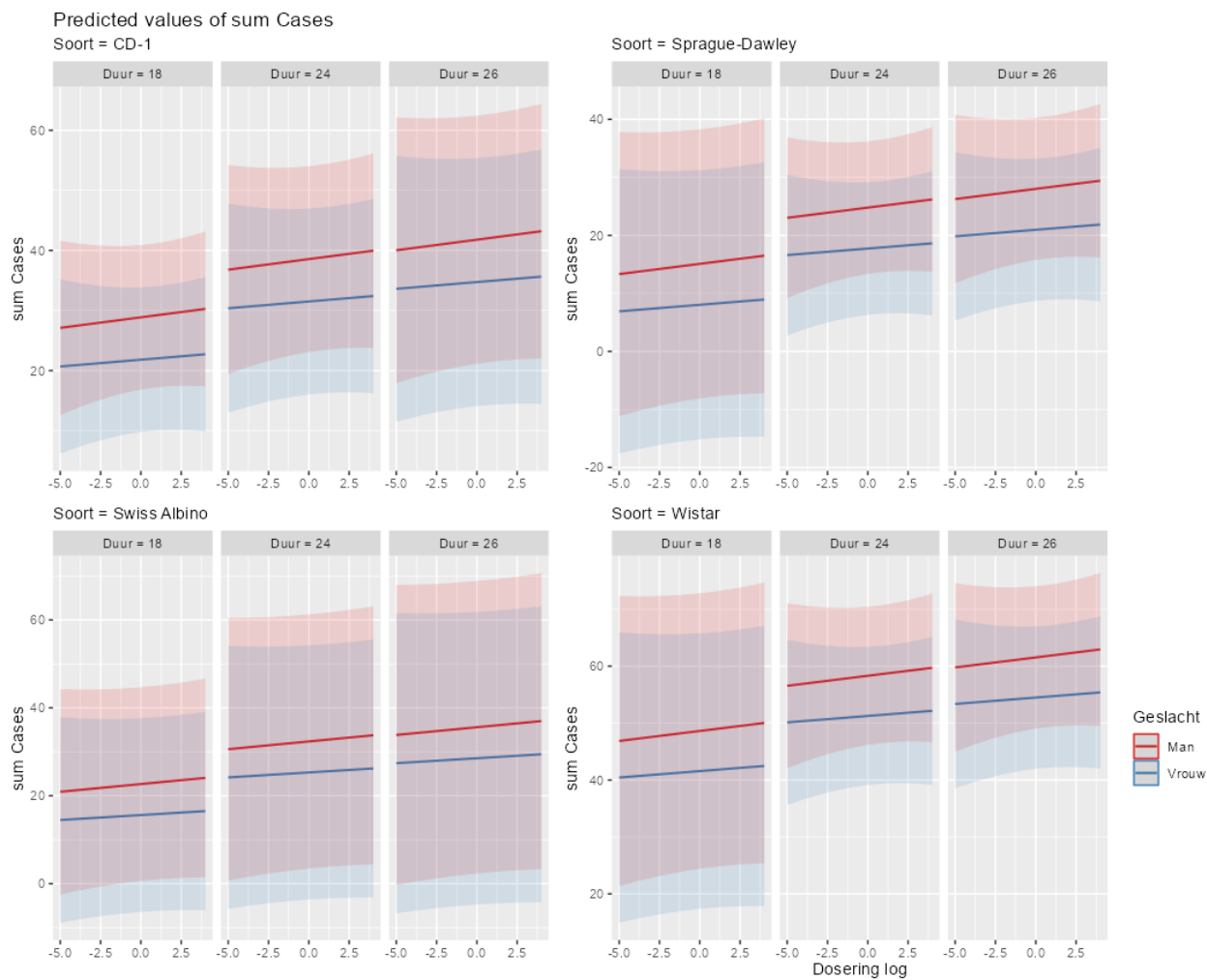
Figuur 94. Voorspellingen vanuit het model per geslacht, soort en duur. De relatie is duidelijk lineair gemodelleerd, maar de nulhypothese (coëfficiënt=0) kan niet worden vervangen. Daarvoor zijn de onzekerheidsbanden te groot.
