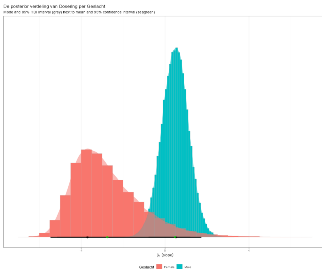
Figuur 148. De posterior verdeling van de parameter Dosering voor mannen en vrouwen.
